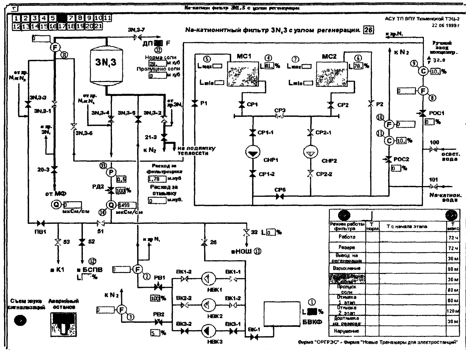
Рисунок 7 – Видеокадр На-катионитного фильтра
