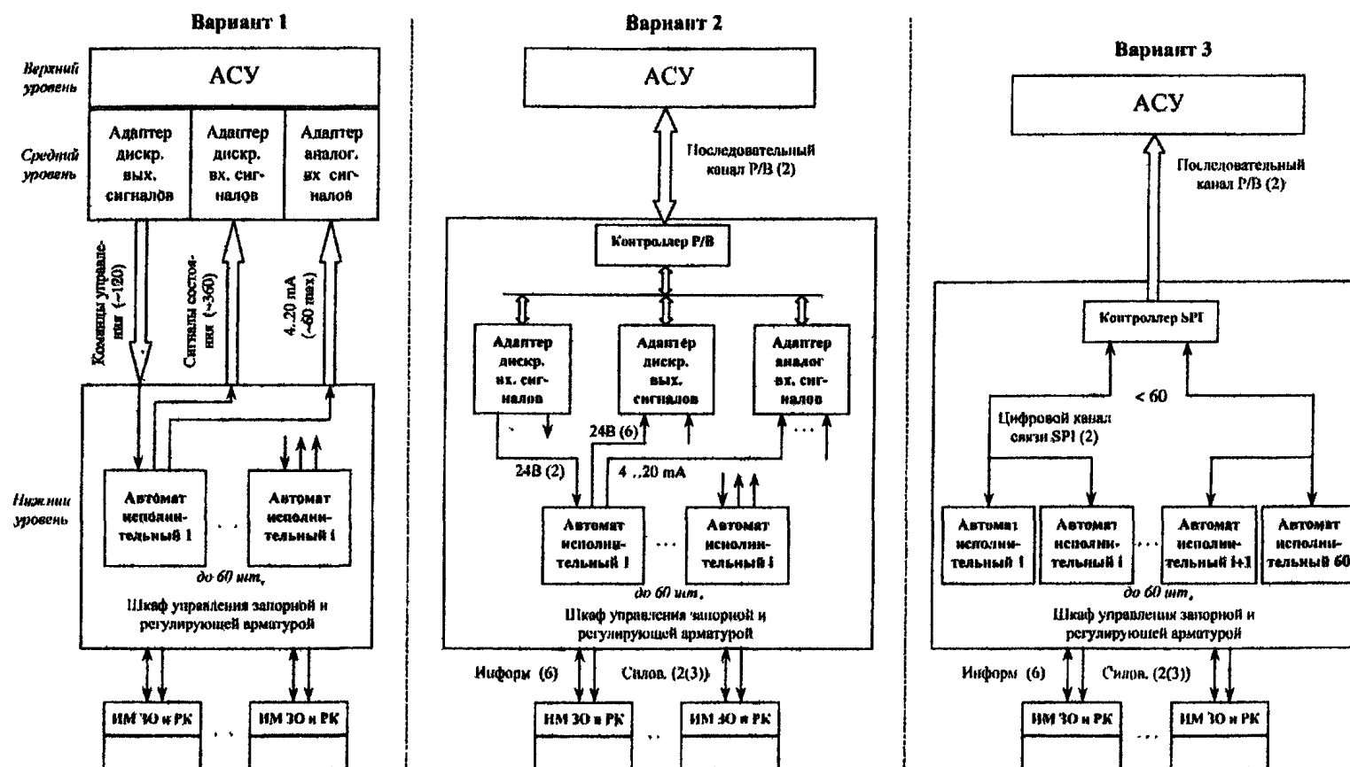
Рисунок 2 – Структурная схема АСУ ТП, нижний уровень которой выполнен на базе электроприводов типа МЭО, МРО с блоками управления АИ (3 варианта)
