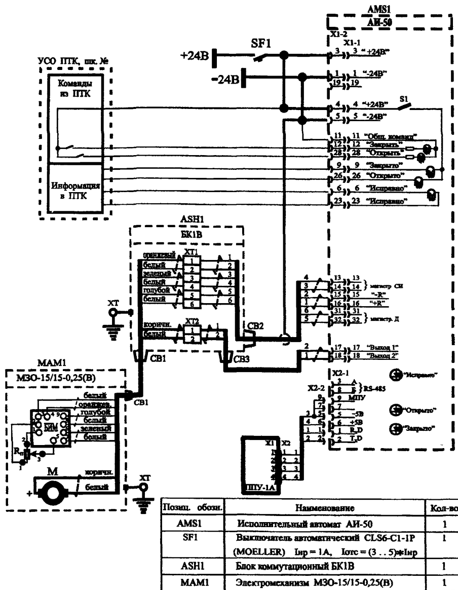
Рисунок Б.4 – Управление электромеханизмом М30-15/15-0,25(В) с АИ-50
