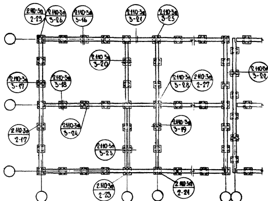
ПРИ ПРОДОЛЬНЫХ НЕСУЩИХ СТЕНАХ КРУПНОПАНЕЛЬНЫЕ ЗДАНИЯ
