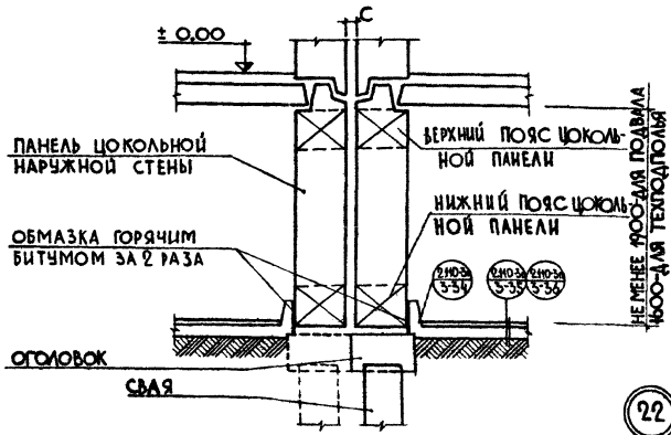
ДЕФОРМАЦИОННЫЙ ШОВ
