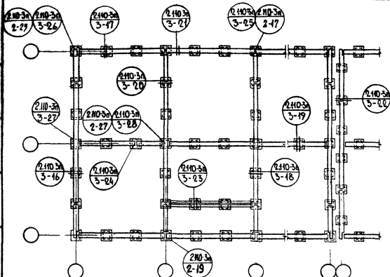
ПРИ ПОПЕРЕЧНЫХ НЕСУЩИХ СТЕНАХ
