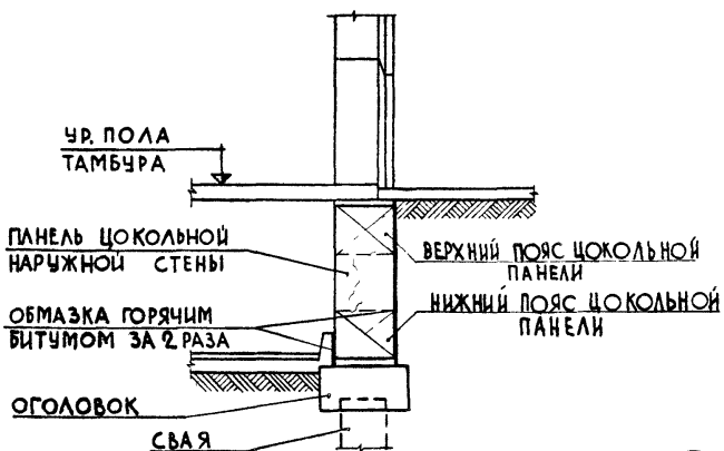
ПОД НАРУЖНЮЮ СТЕНУ
