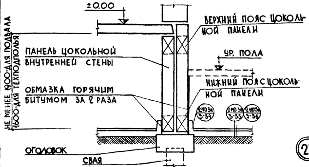
ПОД ВНУТРЕНнюю ВЕНТИЛЯЦИОННУЮ СТЕНУ
