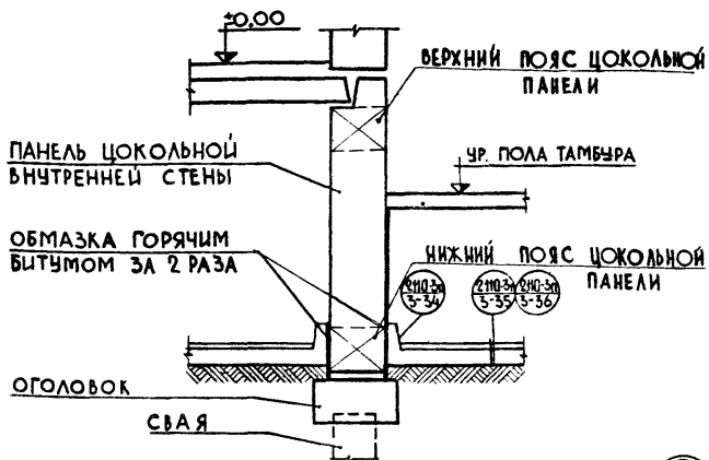
ПОД ВНУТРЕННЮЮ СТЕНУ
