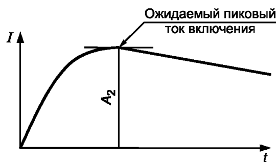
Рисунок 7b — Калибровка испытательной цепи для постоянного тока
