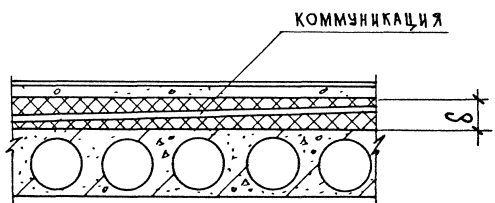
Рис. 2. Прокладка коммуникации в полах с засыпным утеплителем
