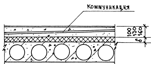
Рис. 1. Прокладка коммуникаций в полах с жестким утеплителем
