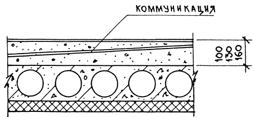
Рис. 3. Прокладка коммуникаций в полах с утеплителем под перекрытием
