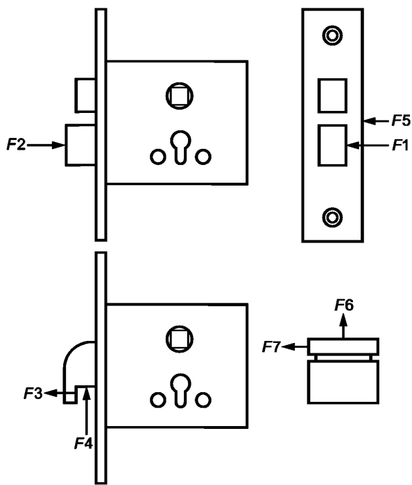
Рисунок 1 — Точки приложения сил, воздействующих на механизм замка
