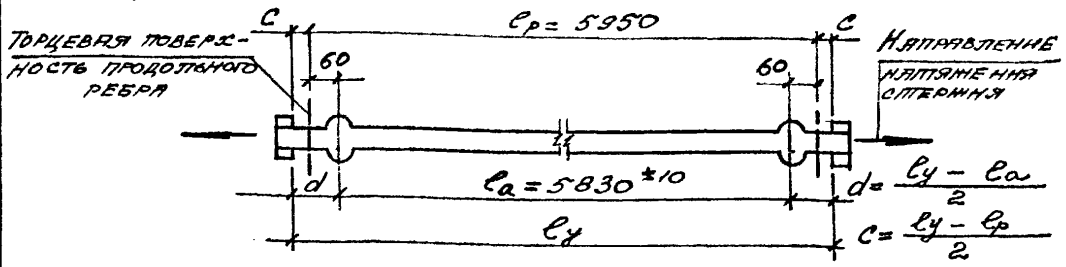
Рис. 2 Натягиваемый стержень с временными концевыми анкерами
