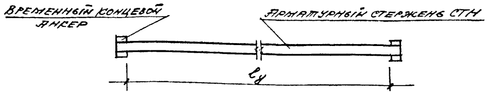
Рис. 2 Натягиваемый стержень с временными концевыми анкерами
