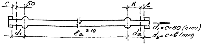
Рис. 3 Натягиваемый стержень с временными концевыми и постоянными анкерами (до его натяжения)
