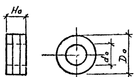
Технические данные Таблица 2 по заготовкам для постоянных анкеров-обжатых шайб
