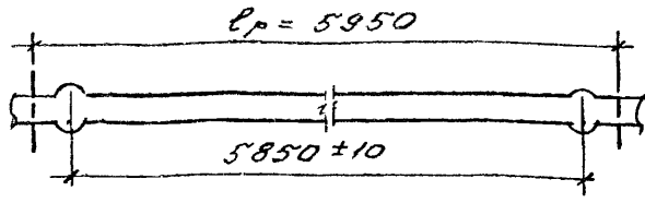
Рис. 4 Проектное положение постоянных анкеров на натянутом стержне (после его натяжения)
