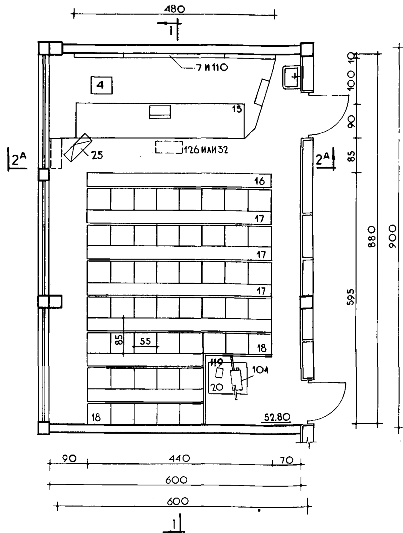
ВАРИАНТ №2 ПЛАН
