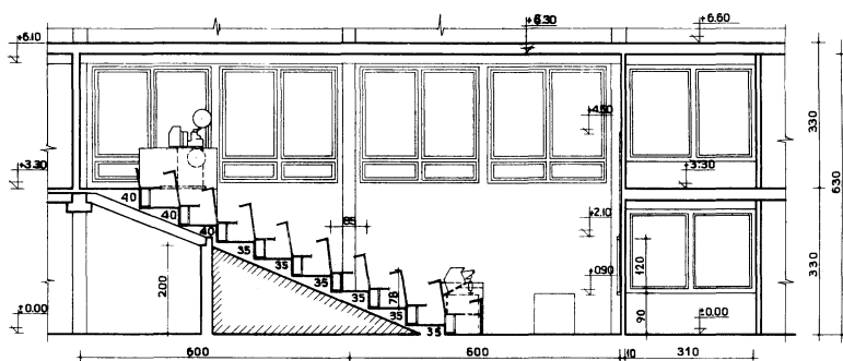
РАЗРЕЗ 2-2
