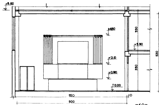
РАЗРЕЗ 2-2
