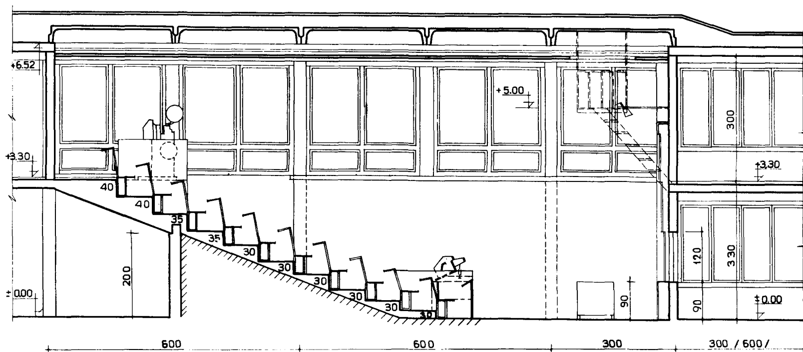
РАЗРЕЗ 1-1
