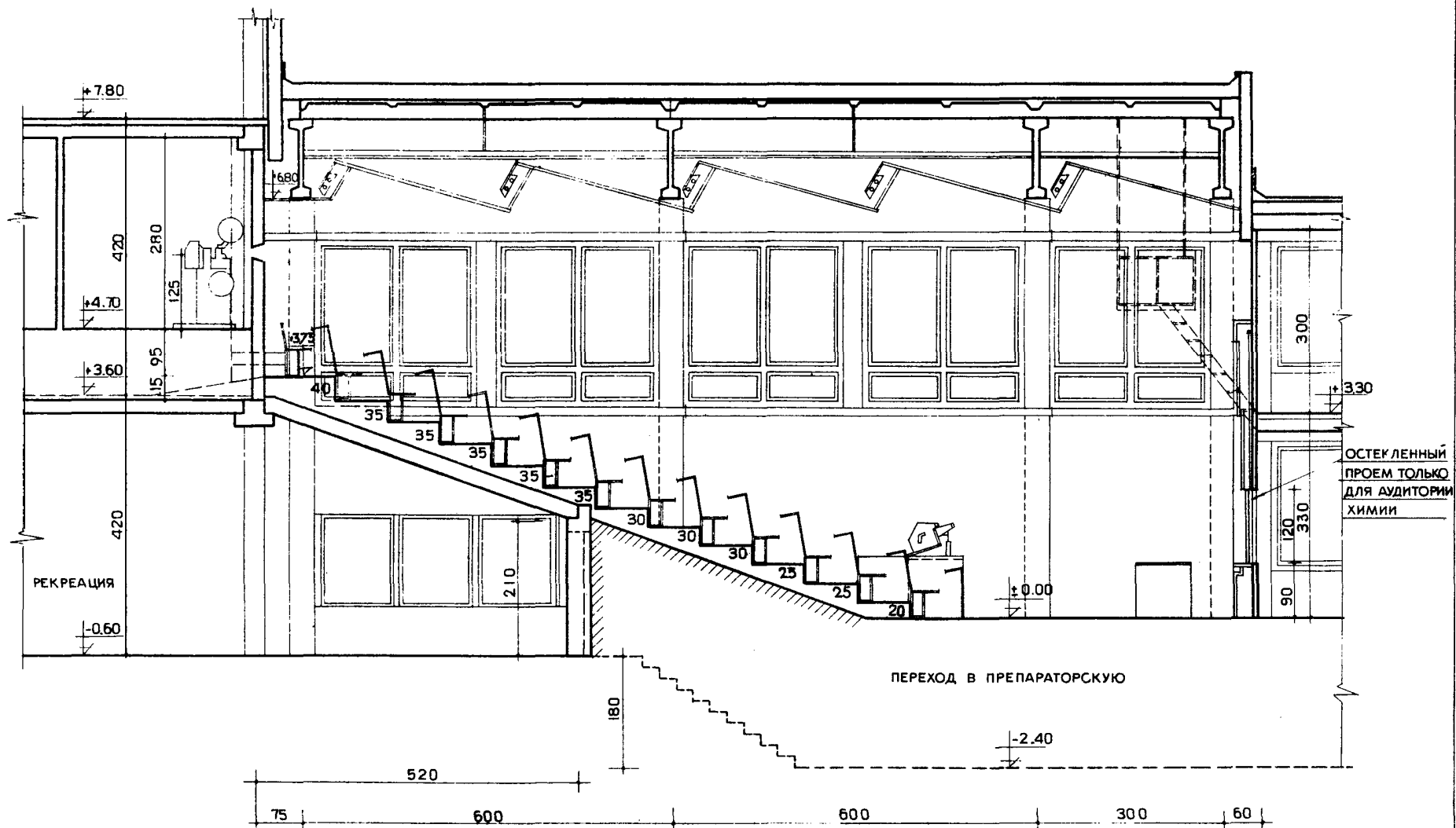
РАЗРЕЗ 2-2
