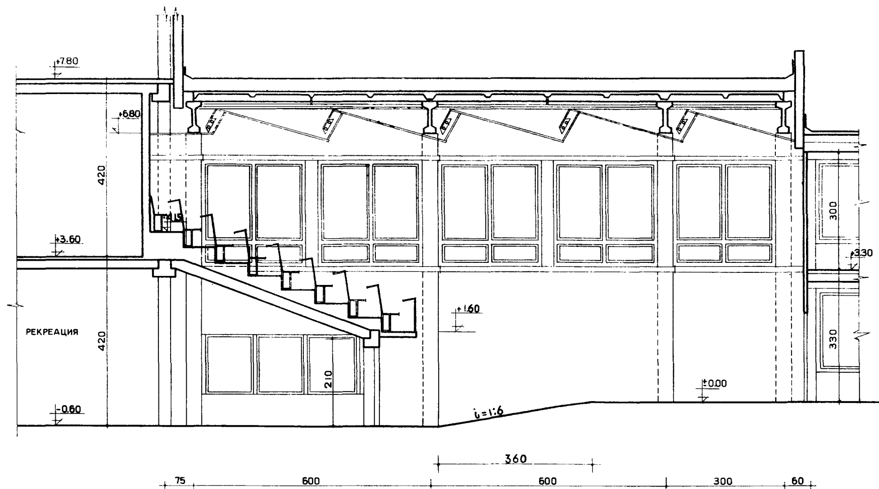
РАЗРЕЗ 3-3
