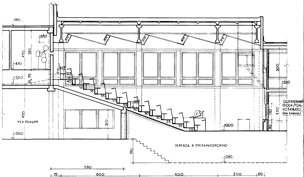
РАЗРЕЗ 2-2
