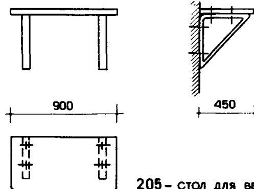
205-СТОЛ ДЛЯ ВЕСОВ
