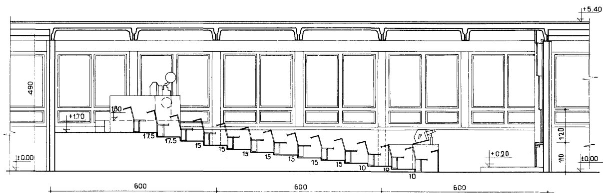
АУДИТОРИЯ тип III-200 РАЗРЕЗ 1-1
