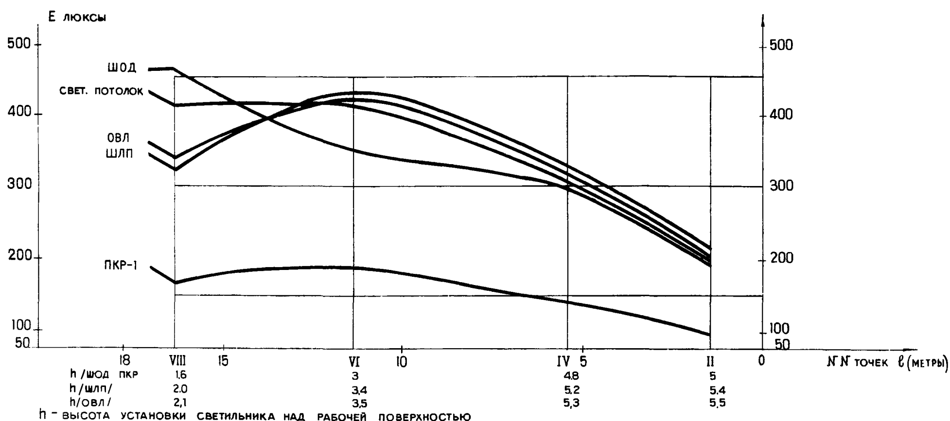
ХАРАКТЕРИСТИКИ ОСВЕТИТЕЛЬНЫХ УСТАНОВОК АУДИТОРИИ НА 200 МЕСТ
