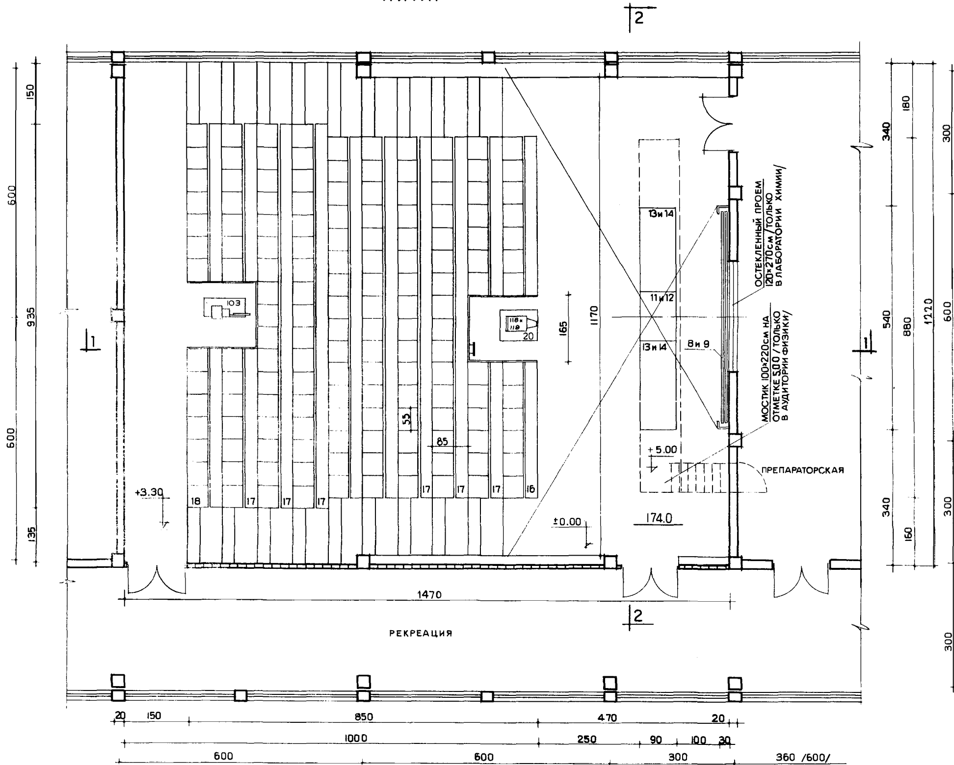
ПЛАН
