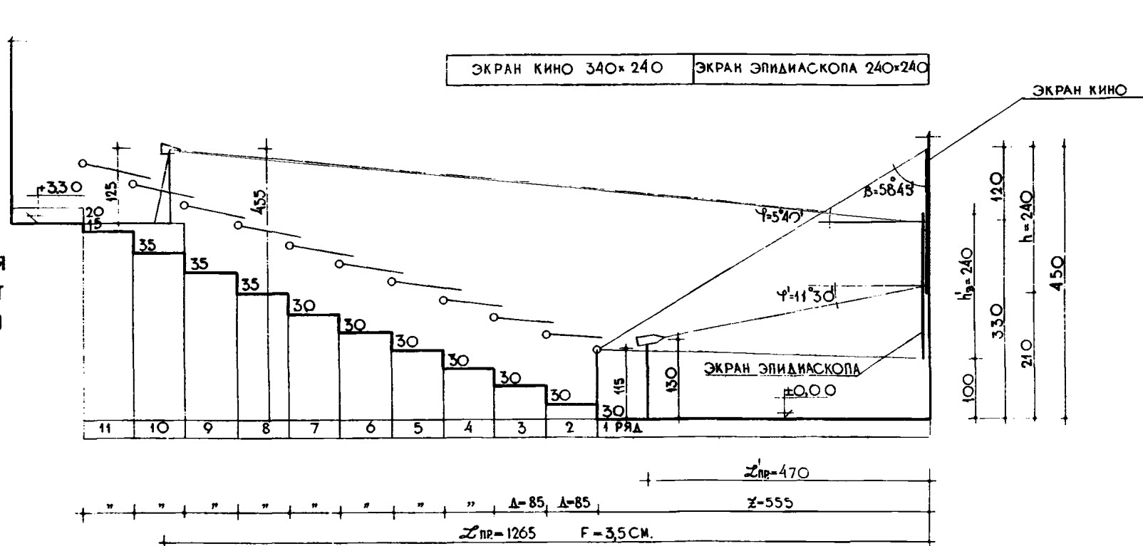
АУДИТОРИЯ НА 150 МЕСТ ТИП I-150
