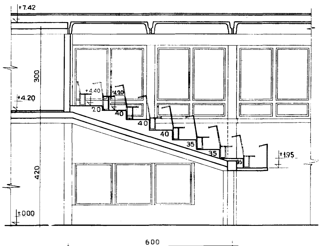
РАЗРЕЗ 2-2
