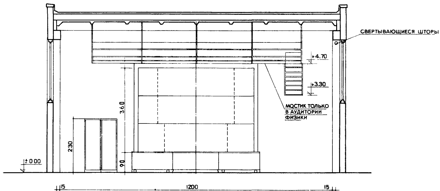
РАЗРЕЗ 3-3
