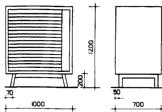
206-ТАБУРЕТ ЛАБО- РАТОРНЫЙ ВЫ- СОКИЙ
