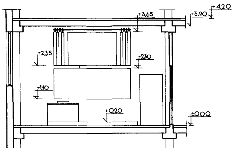
РАЗРЕЗ 2-2
