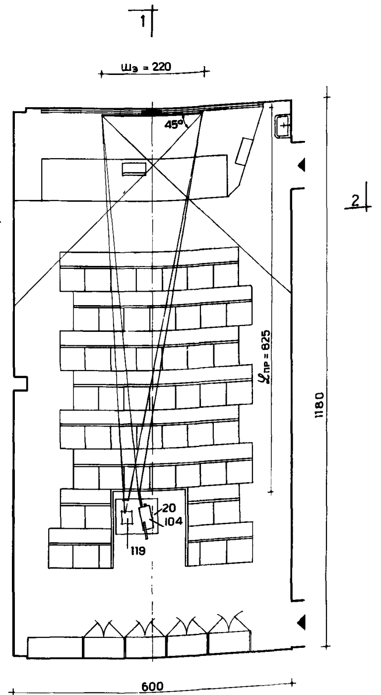
ВАРИАНТ 1. ПЛАН
