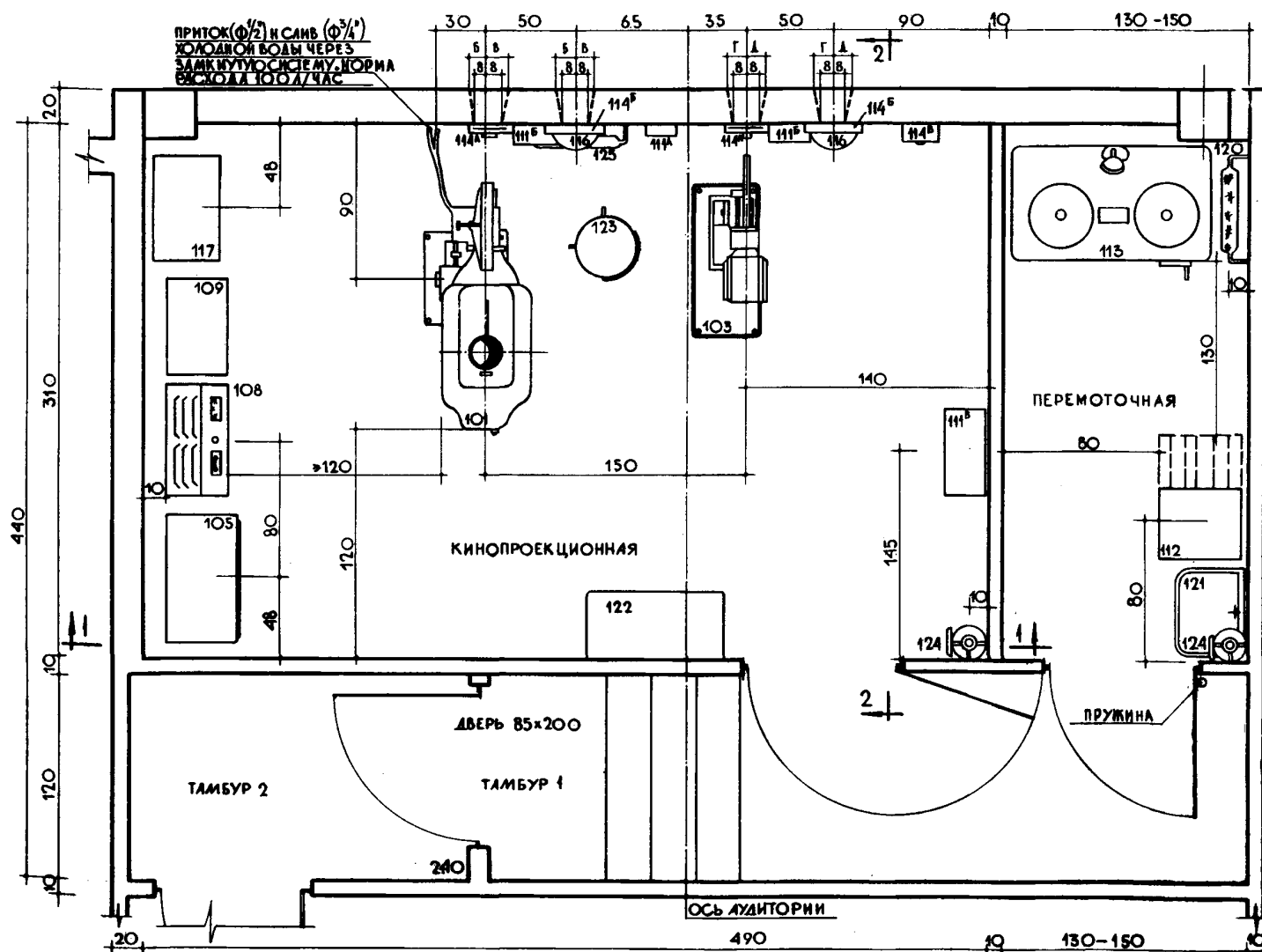
ПЛАН
