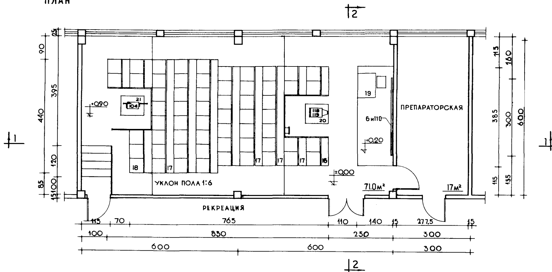
ПЛАН
