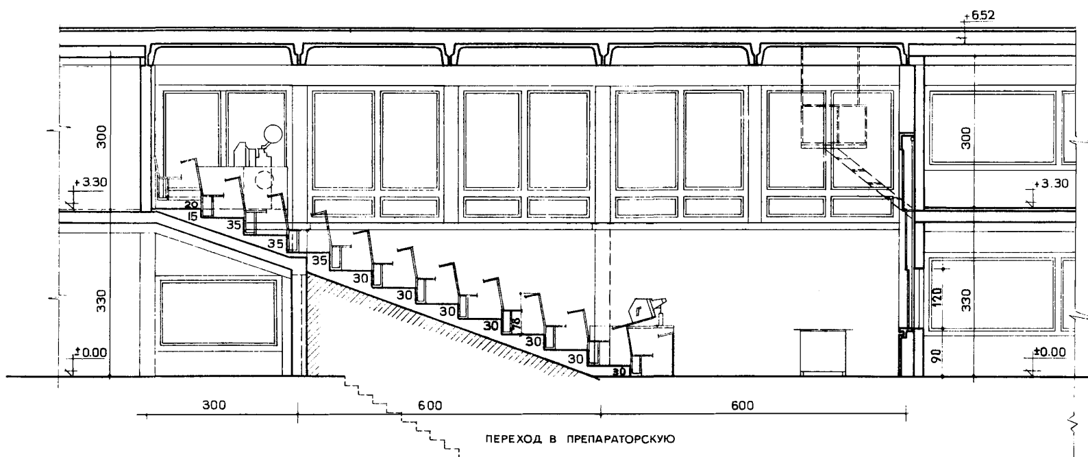
РАЗРЕЗ 2-2
