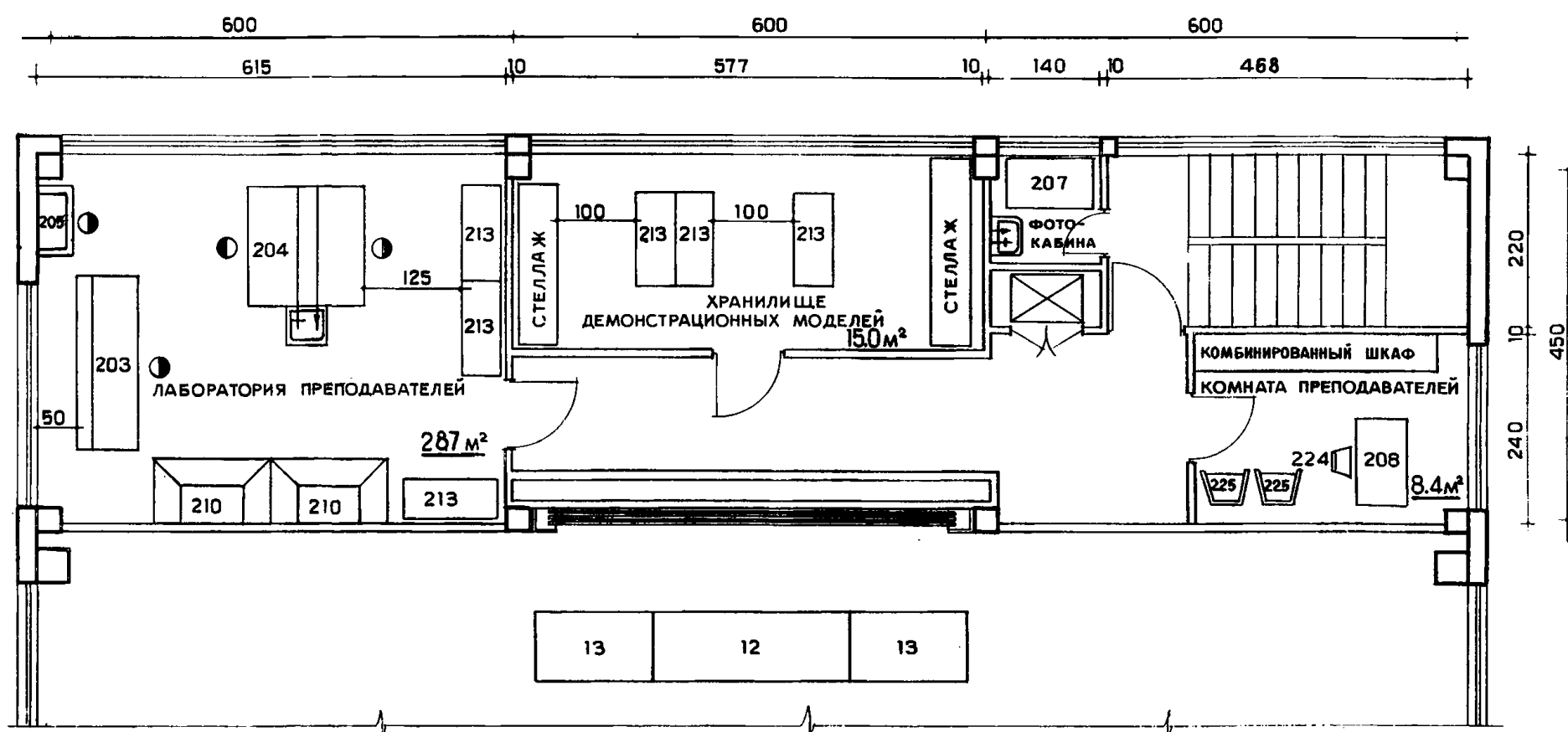
ПЛАН 2-ГО ЭТАЖА
