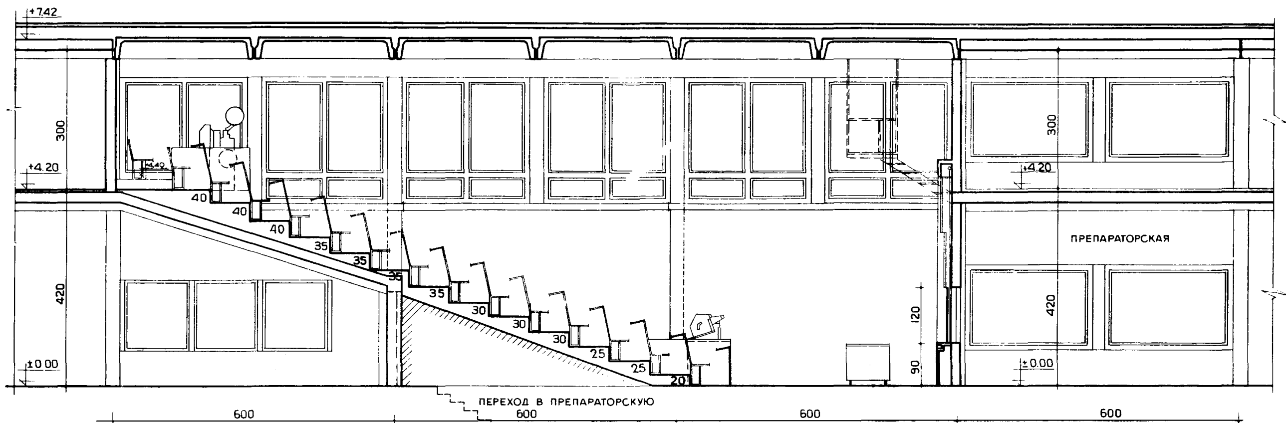
РАЗРЕЗ 2-2
