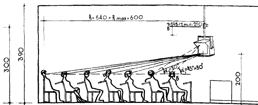
РАЗРЕЗ 1-1
