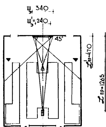
ТИП I-150 СХЕМА ПЛАНА
