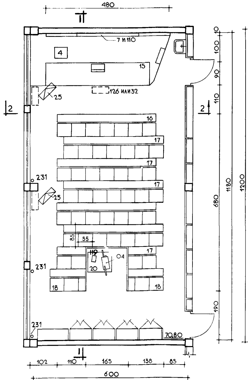
ВАРИАНТ №1 ПЛАН
