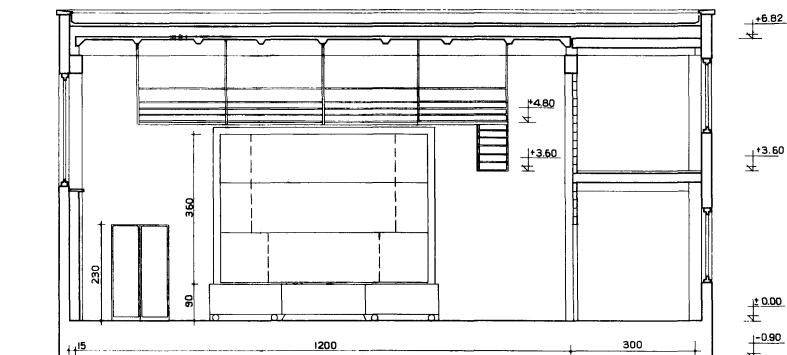
РАЗРЕЗ 2-2
