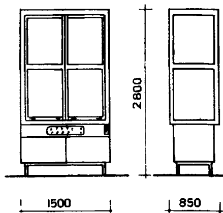
210 ШКАФ ВЫТЯЖНОЙ.
