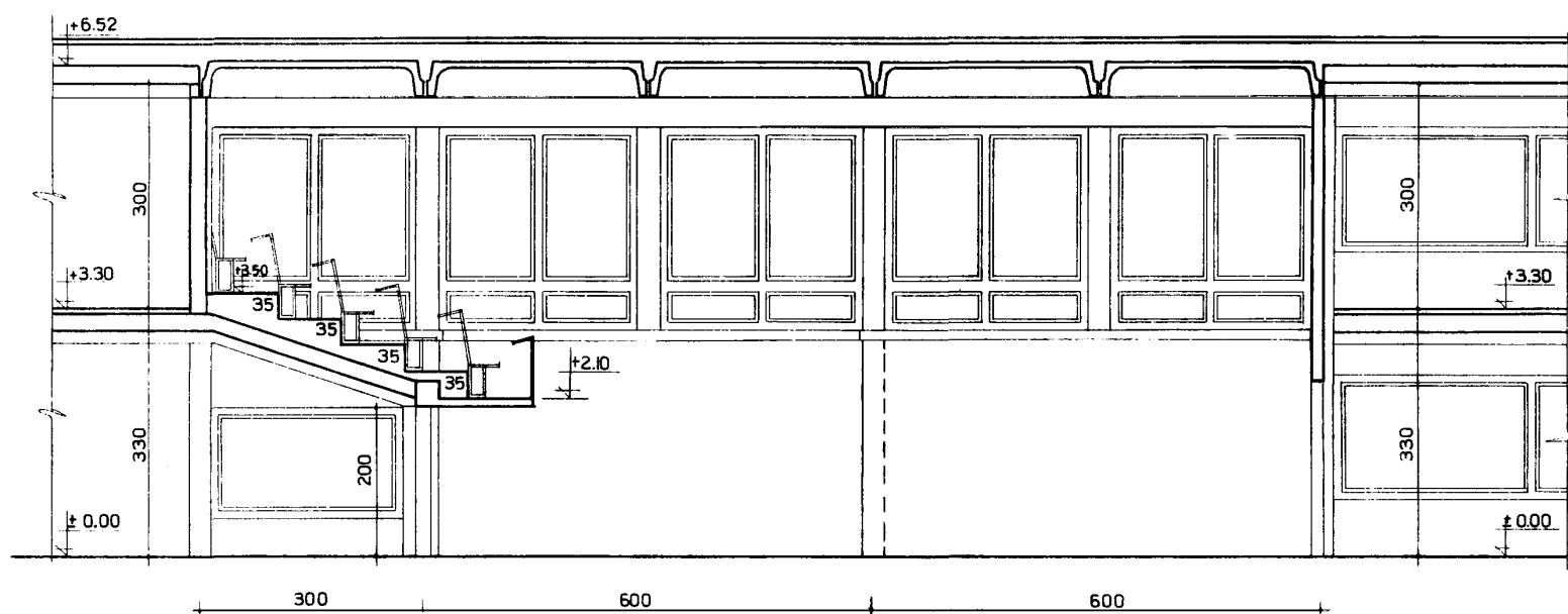
РАЗРЕЗ 2-2
