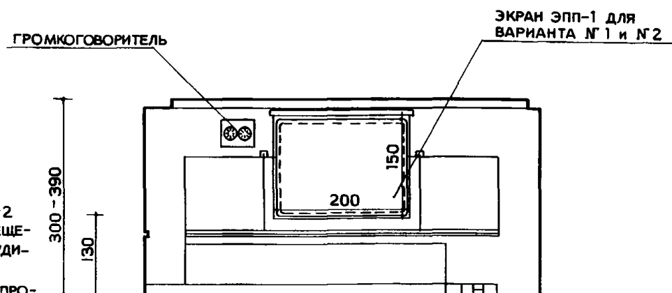
СОВМЕЩЕННЫЙ РАЗРЕЗ 2-2 и 2 А -2 А
