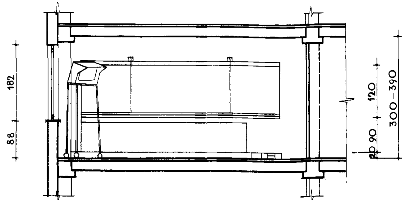
СОВМЕЩЕННЫЙ РАЗРЕЗ 2-2 и 2 А -2 А
