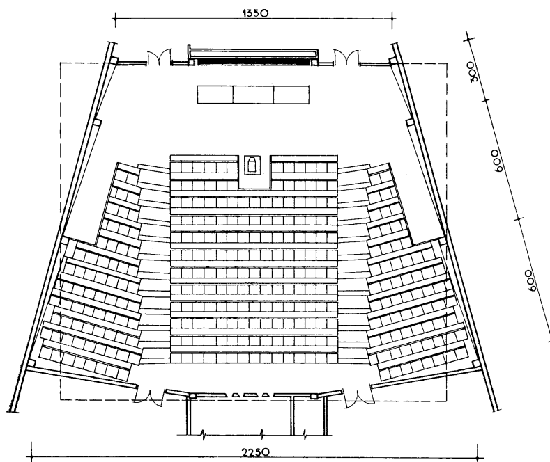
ВАРИАНТ ТРАПЕЦИЕДАЛЬНЫХ ГАБАРИТОВ ПЛАНА
