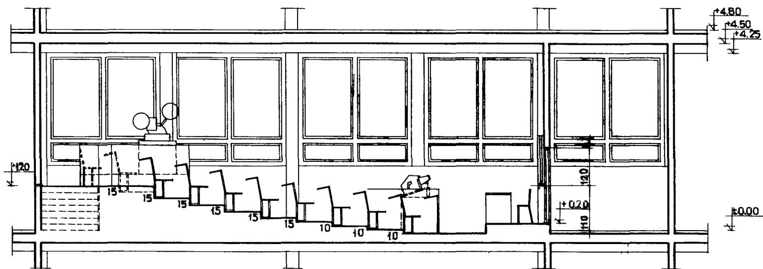
РАЗРЕЗ 2-2
