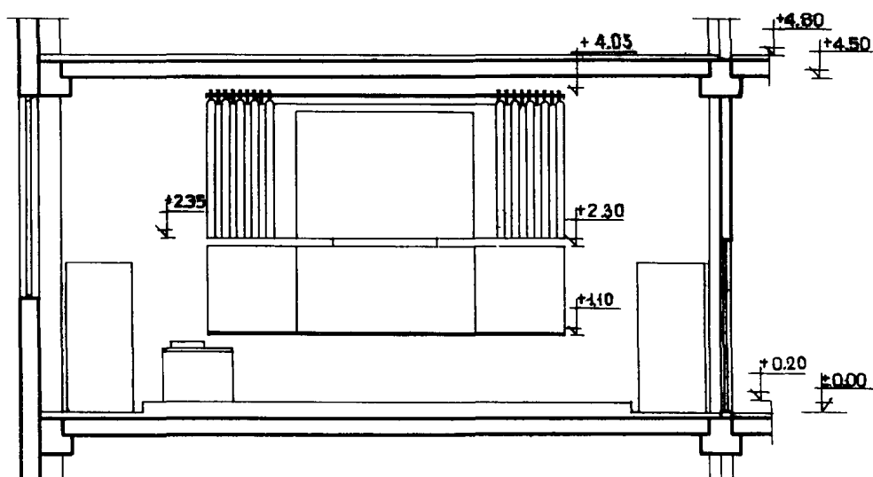
РАЗРЕЗ 2-2
