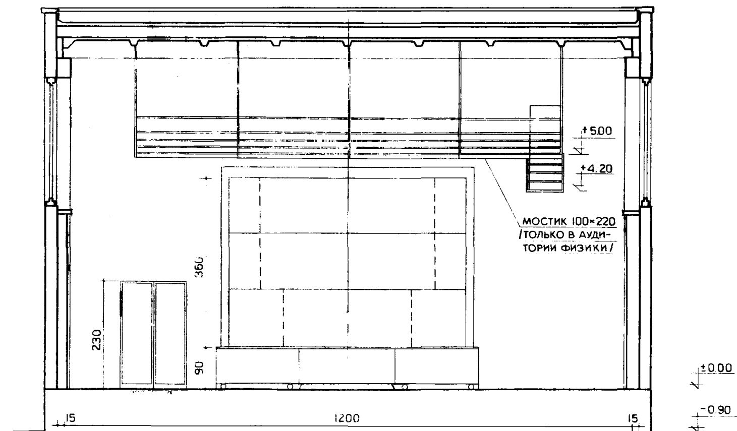
РАЗРЕЗ 3-3
