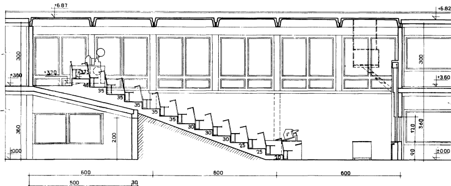
РАЗРЕЗ 1-1
