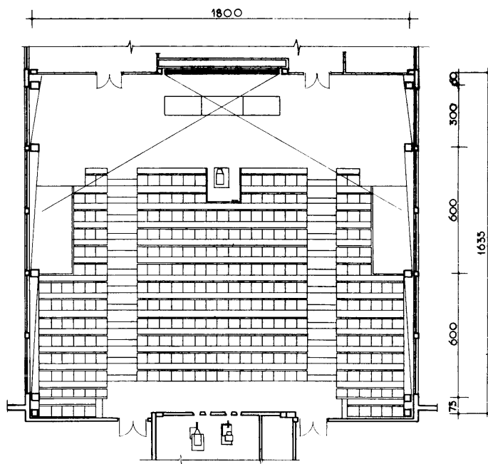
ВАРИАНТ ТРАПЕЦИЕДАЛЬНЫХ ГАБАРИТОВ ПЛАНА
