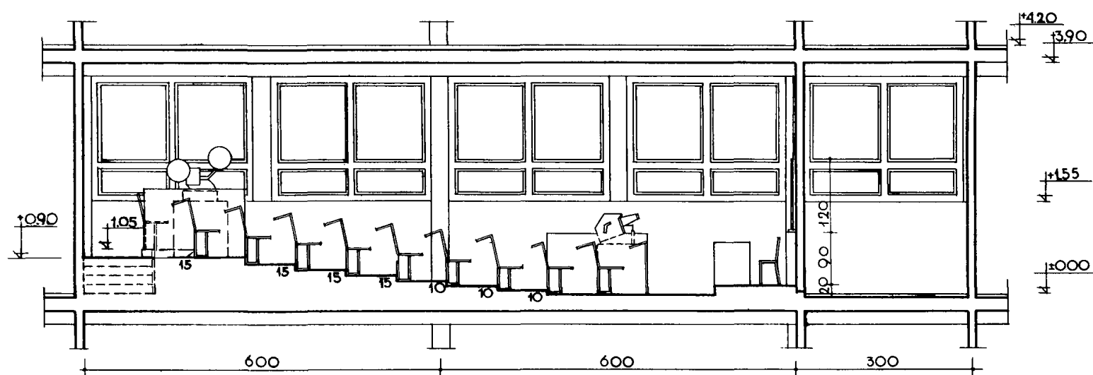
РАЗРЕЗ 1-1
