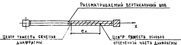
Рис.8 Схематический план сечения диафрагмы к определению сдвигающих сил в вертикальных швах (заштрихована условно отсеченная часть диафрагмы).
