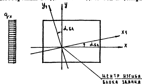
Рис. 10. Схема приложения односторонней нагрузки q_x вдоль оси X
