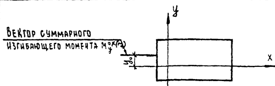
Рис.6. Схема приложения суммарного изгибающего момента M_{y, \kappa}^{0, \kappa}(r_2) к блоку здания
