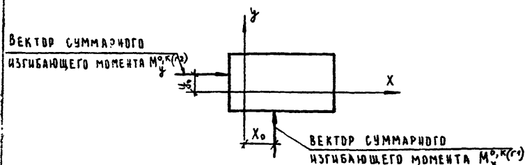
Рис.7. Схема приложения суммарных изгибающих моментов M_{x, \kappa}^{0, \kappa}(r_1) и M_{y, \kappa}^{0, \kappa}(r_2) к блоку здания.
