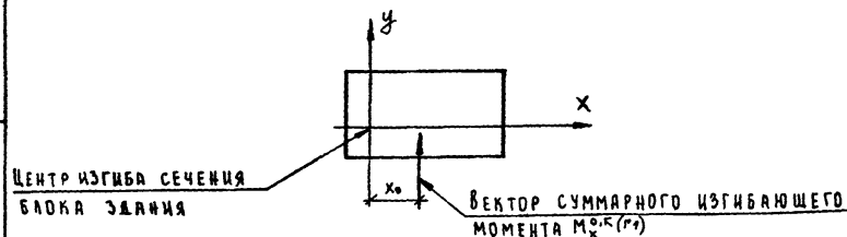
Рис.5. Схема приложения суммарного изгибающего момента M_x^{o,k(r1)} к блоку здания.
