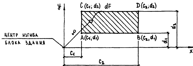
Рис. 4 Схема для определения интеграла \int_{F_{\text{БЛ}}} \rho^2 dF , вычисляемого по формуле (6.15).
