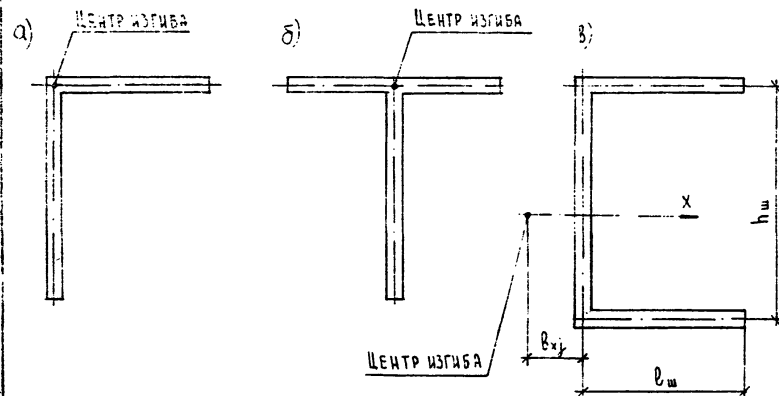
Рис.2. Схемы расположения центров изгиба диафрагм различных очертаний в плане: а) уголкового; б) таврового; в) [ образного.
