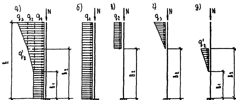
Рис. 9. Схема разделения эпюры интенсивности суммарной нормативной горизонтальной нагрузки q на составляющие q_1 , q_2 , q_3 и q'_2 .
