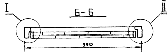
Дверное полотно ДП.13.01.00.00.СБ
