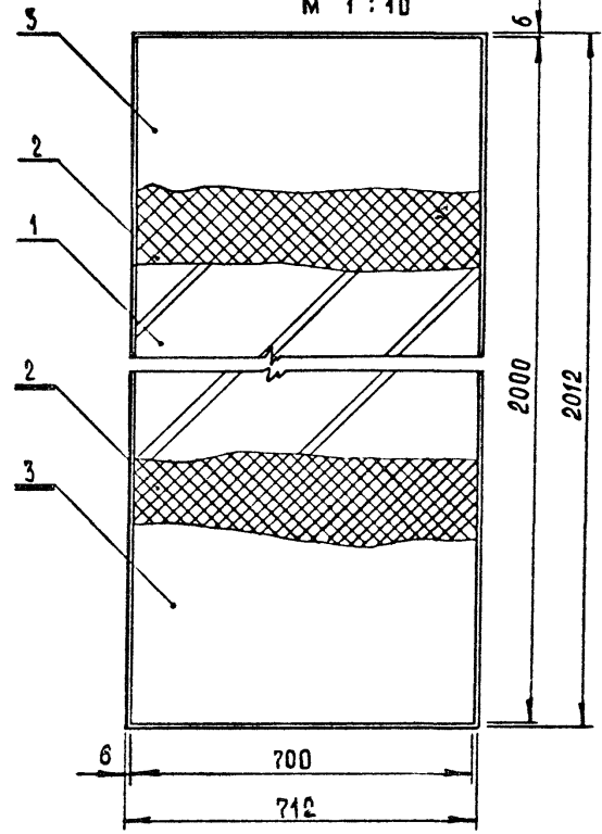
ДВЕРНОЕ ПОЛОТНО ДП209.01.00.00 СБ М 1:10
