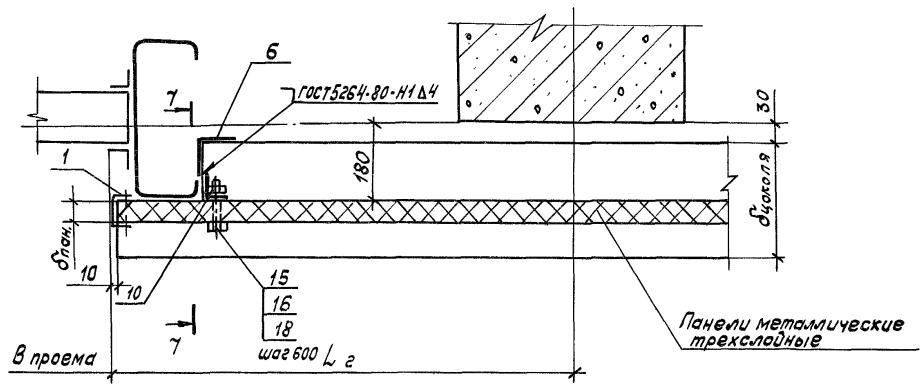
6-6 лист 1
