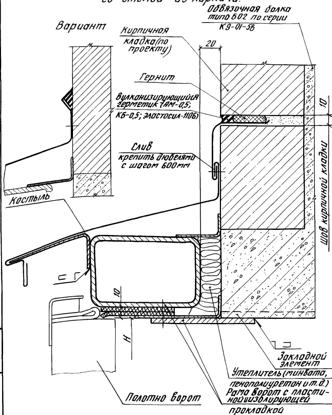
Рис. 14. Пример сопряжения ригеля рамы с стеной из кирпича.
