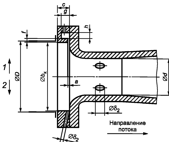
1 — с кольцевой щелью; 2 — с отдельным отверстием
