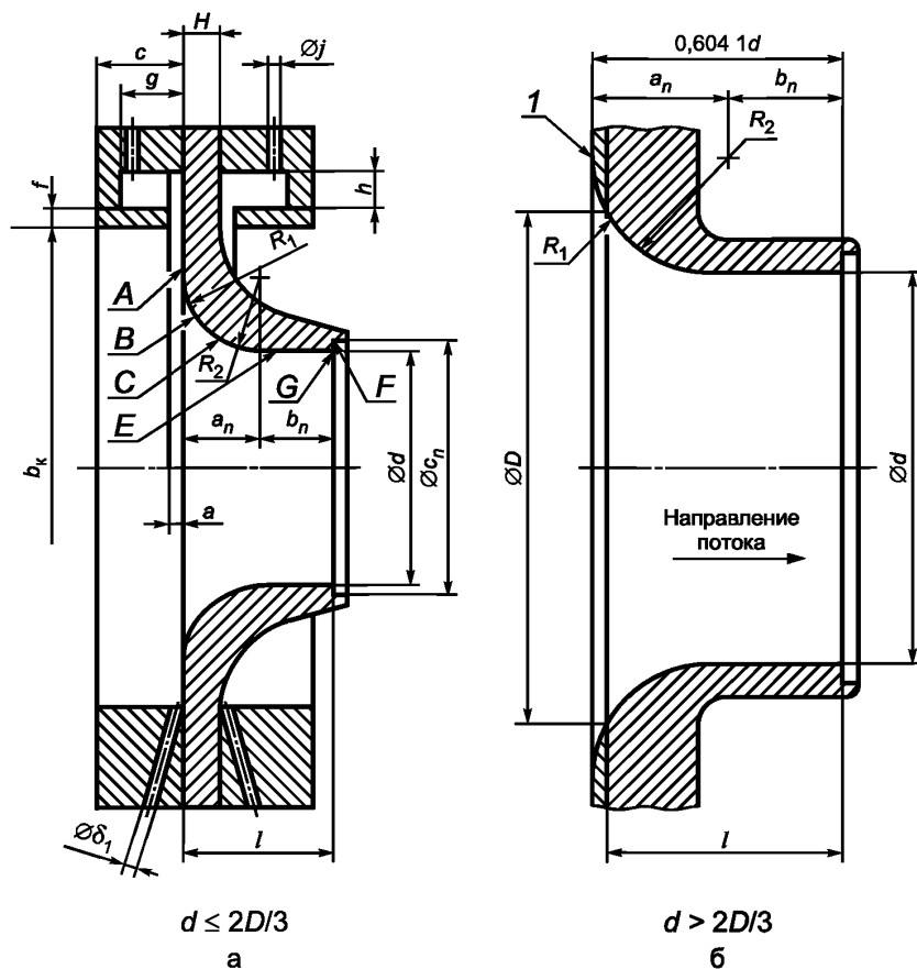
Рисунок 1 — Сопло ИСА 1932
