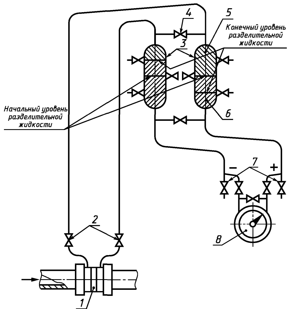
1 — СУ; 2 — кран СУ; 3 — разделительный сосуд; 4 — уравнильный вентиль; 5 — измеряемый газ; 6 — разделительная жидкость; 7 — продувочный вентиль; 8 — ППД
