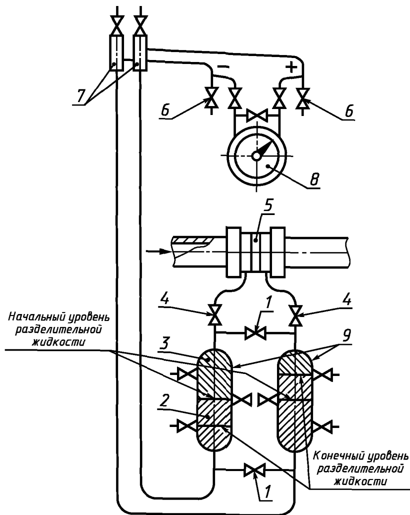
1 — уравнительный вентиль; 2 — разделительная жидкость; 3 — измеряемая жидкость; 4 — кран; 5 — СУ; 6 — продувочный вентиль; 7 — газосборник; 8 — ППД; 9 — разделительный сосуд
