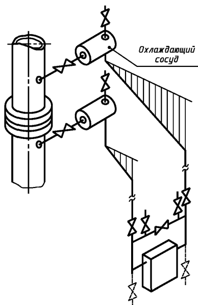
Рисунок Г.17 — Вертикальный трубопровод
