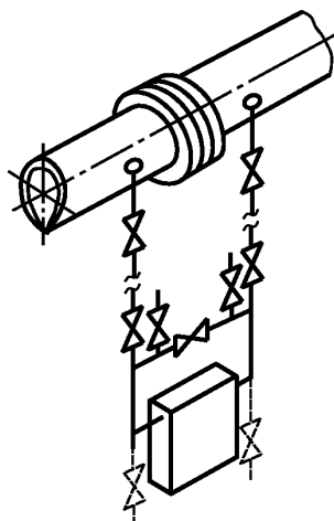
Рисунок Г.2 — ППД под трубо- водом
