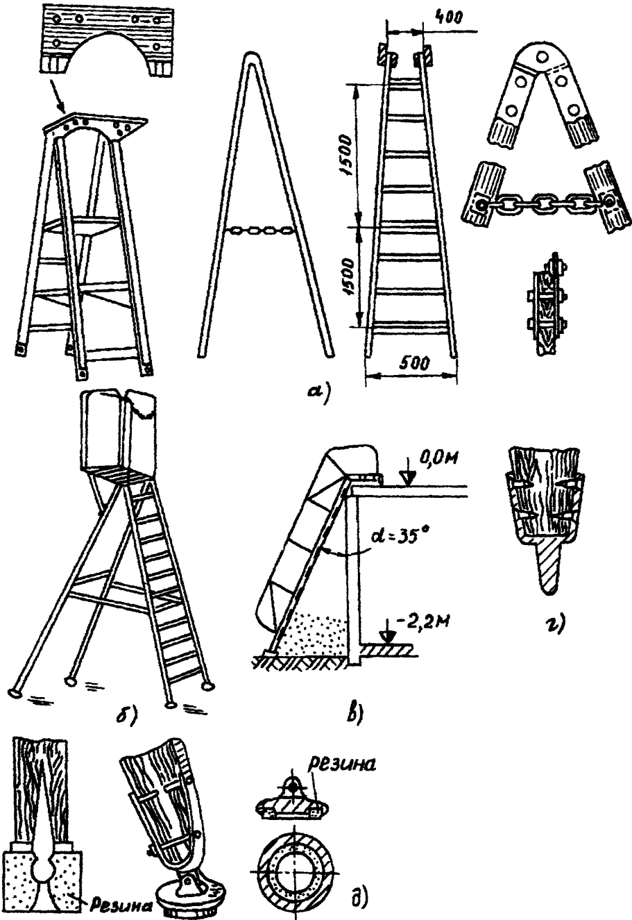
Рис. 5.3. Стремянки:
