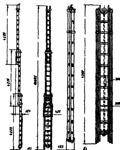
Рис. 5.1. Условное изображение приставной раздвижной лестницы Л-3К:
