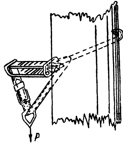
Рис. 6.1. Схема испытания монтерских когтей (P - испытательная нагрузка)
