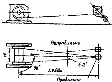
Рис. 4.2. Намотка каната на барабан лебедки
