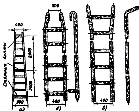
Рис. 5.2. Лестницы одноколенные:
