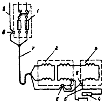
Рис. 7.1. Схема подключения сварочного трансформатора:
