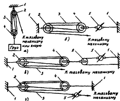
Рис. 4.4. Схема испытания многорольных блоков и полиспастов:
