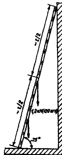
Рис. 5.5. Схема испытания приставной лестницы
