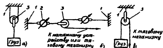
Рис. 4.3. Схема однорольных блоков:
