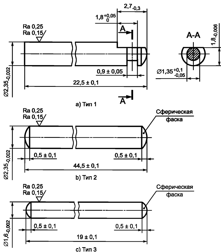
Рисунок 2 — Контрольные оправки
