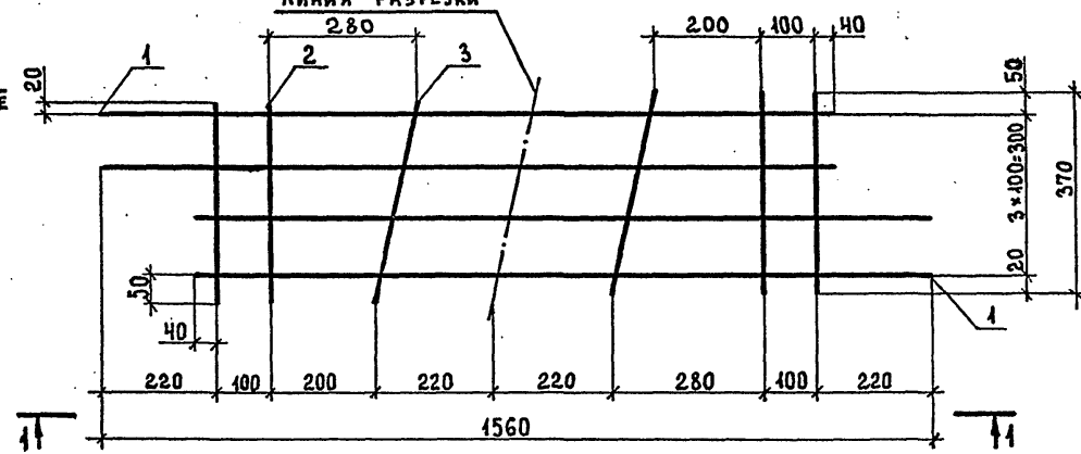
Заготовка для КР4 (КР5)
