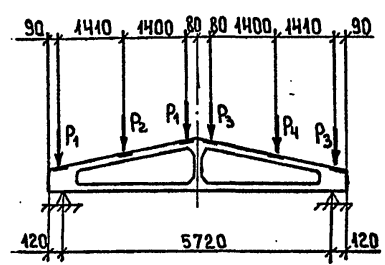
Схема приложения контрольных нагрузок
