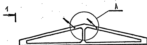
Рис. 1 Строповка ферм при кантовании (выемка из формы)
