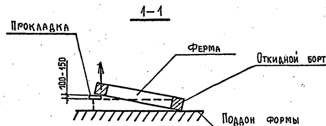
Рис. 1 Строповка ферм при кантовании (выемка из формы)
