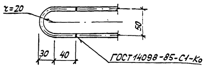
Деталь приварки поз. 4 к поз. 1
