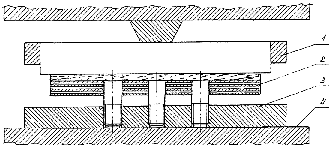
1-опорная планка; 2-образец для испытаний; 3-вилка; 4-опорная площадка испытательной машины
