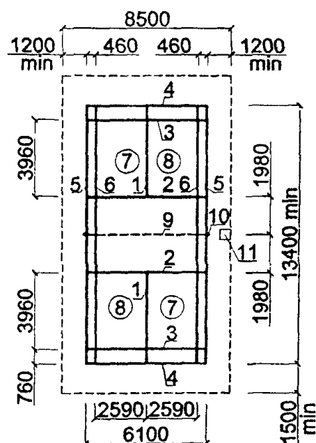
Г. ПЛОЩАДКА ДЛЯ ИГРЫ В БАДМИНТОН
