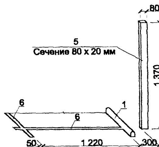
СХЕМА УСТАНОВКИ ФИНИШНОГО СТОЛБА
