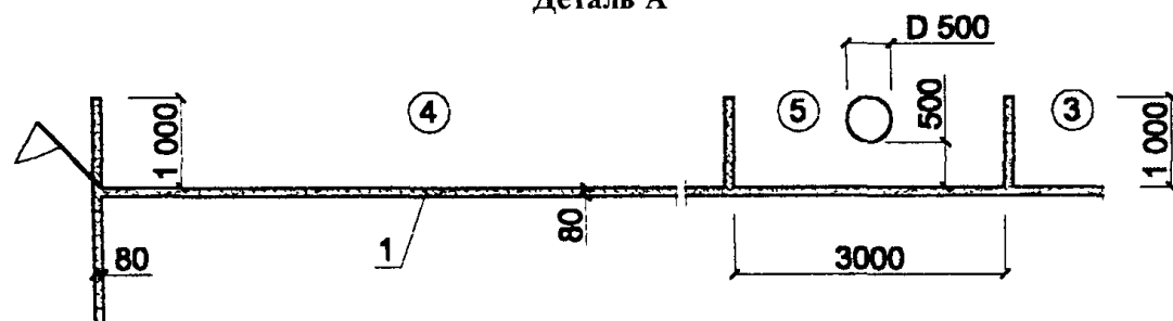
Деталь А
