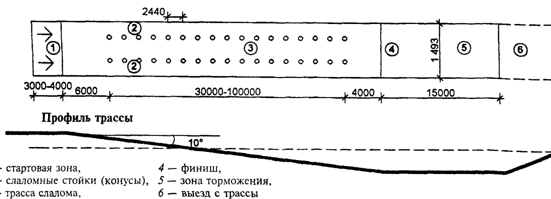
План трассы
