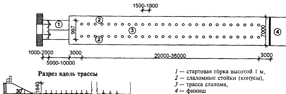
План трассы
