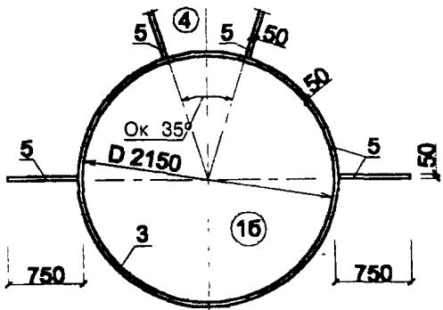
Б. МЕСТО ДЛЯ МЕТАНИЯ ДИСКА
