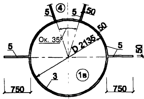
Г. СОВМЕЩЕННЫЕ МЕСТА
