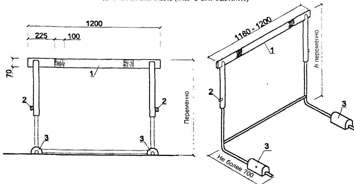
Б. ПЕРЕНОСНОЕ ПРЕПЯТСТВИЕ (БАРЬЕР) ДЛЯ СТИПЛЬ-ЧЕЗА
