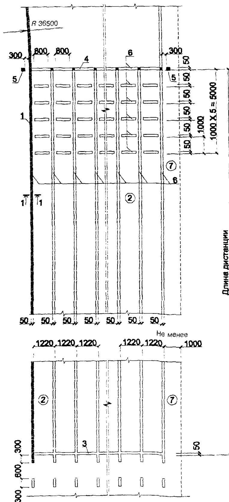
СХЕМА РАЗМЕТКИ ПРЯМОЙ БЕГОВОЙ ДОРОЖКИ
