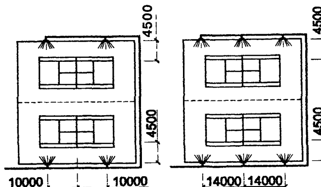
Г. Спаренных теннисных площадок
