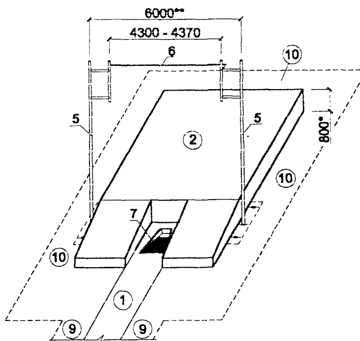
Б. ВАРИАНТ С АЛЬТЕРНАТИВНЫМИ СТОЙКАМИ
