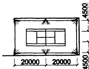
В. Теннисной площадки
