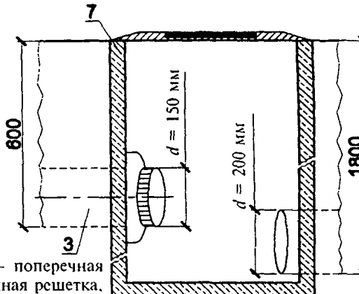
Узел В
