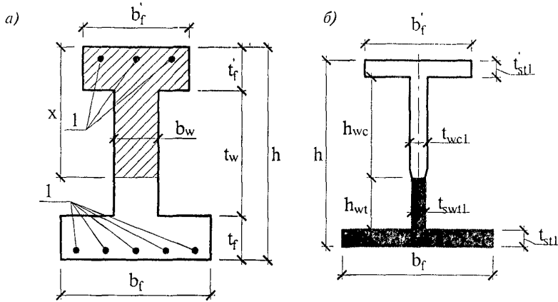
а — сечение сталефибробетонного элемента; б — сечение, приведенное к стальному; I — стержневая арматура Рисунок 7.1 — Схема приведения сечения сталефибробетонных элементов к стальному
