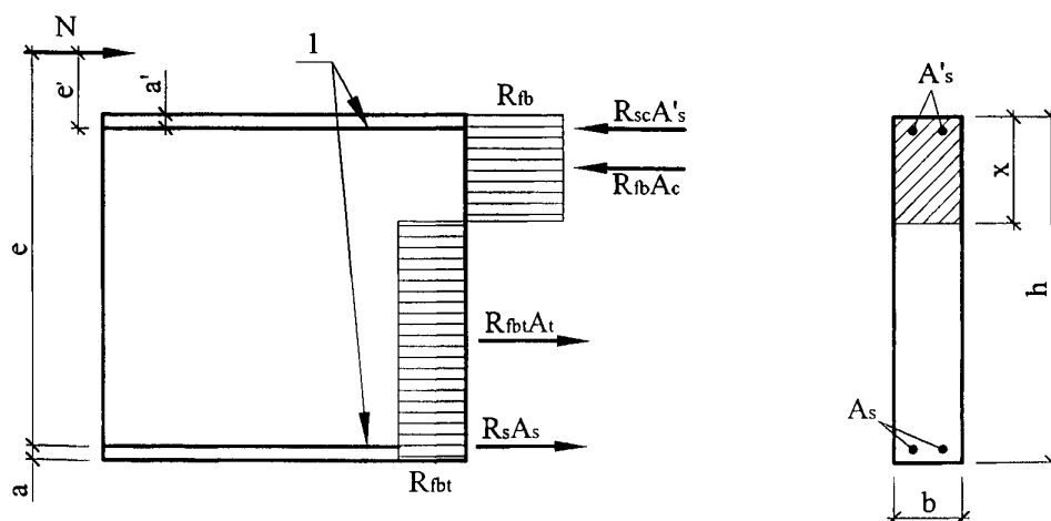
1 — стержневая арматура
