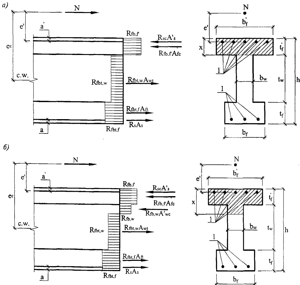
Рисунок 6.6 — Схема усилий и эпюра напряжений во внецентренно сжатых элементах двутаврового сечения при комбинированном армировании
