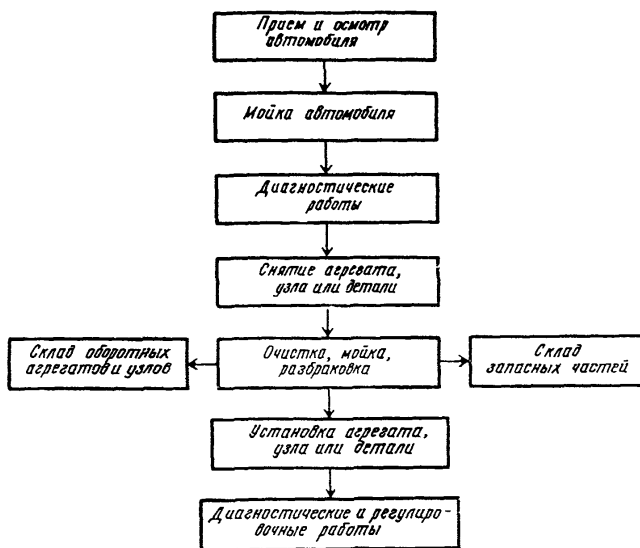
Схема постовых работ по ремонту автомобилей
