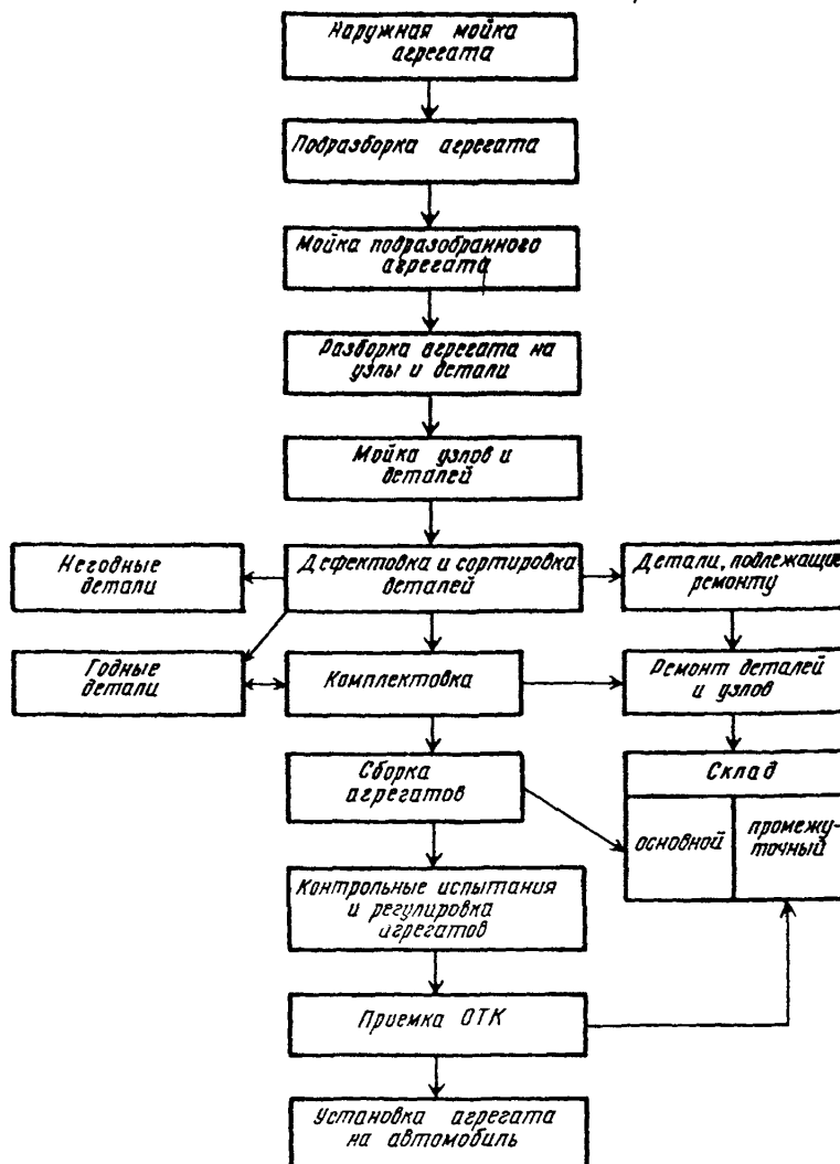
Схема технологического процесса текущего ремонта агрегатов (цеховые работы)
