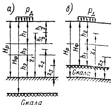
Рис. 3. Схема к определению H_p
