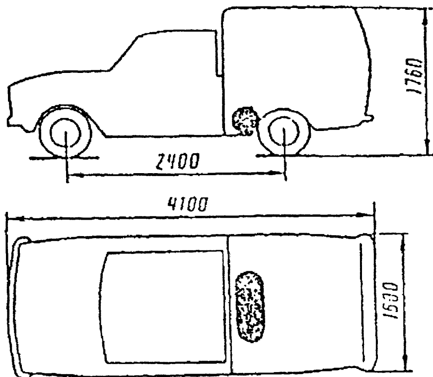
Автомобиль ИЖ-2715.07
