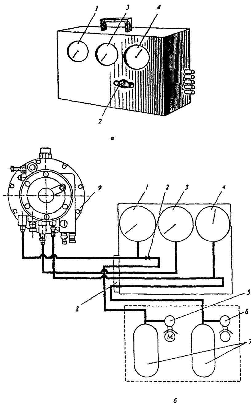
Рис. 6.5. Стенд НПФ «САГА»:
