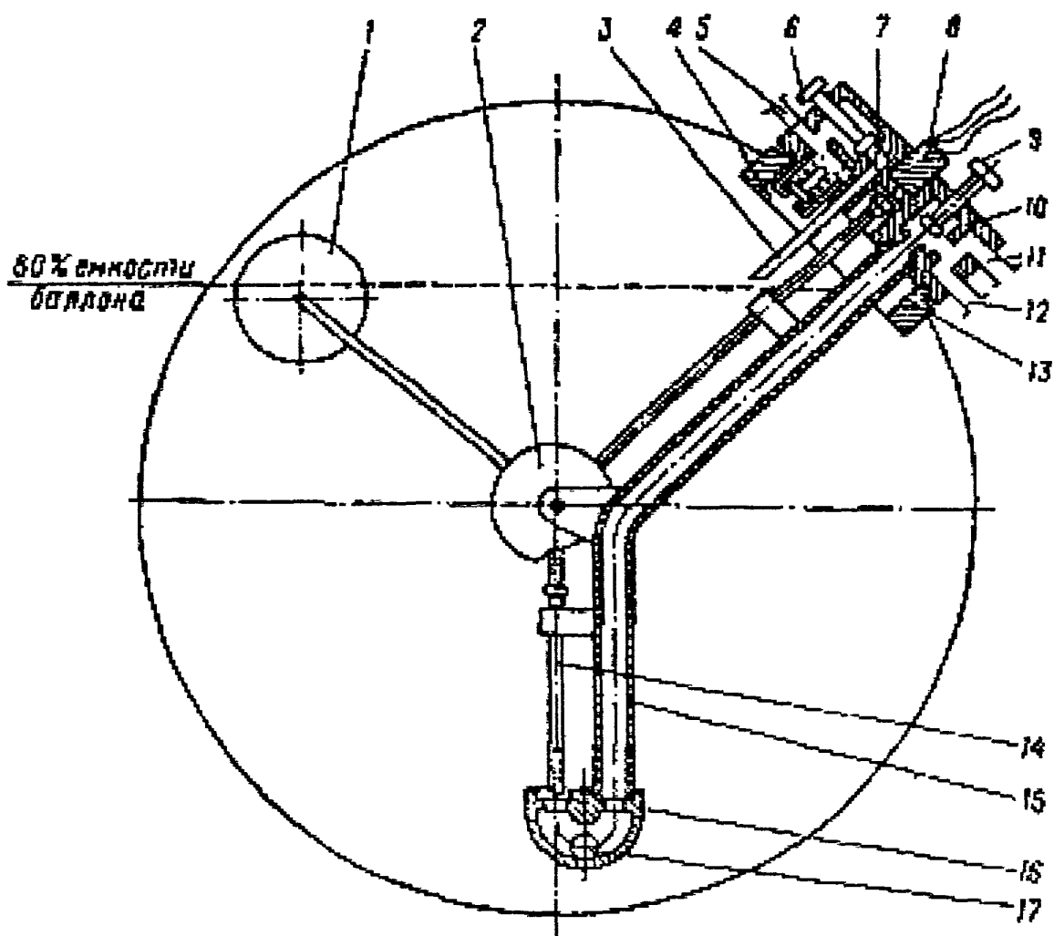
Рис. 3.9. Блок арматуры «САГА - 6»:
