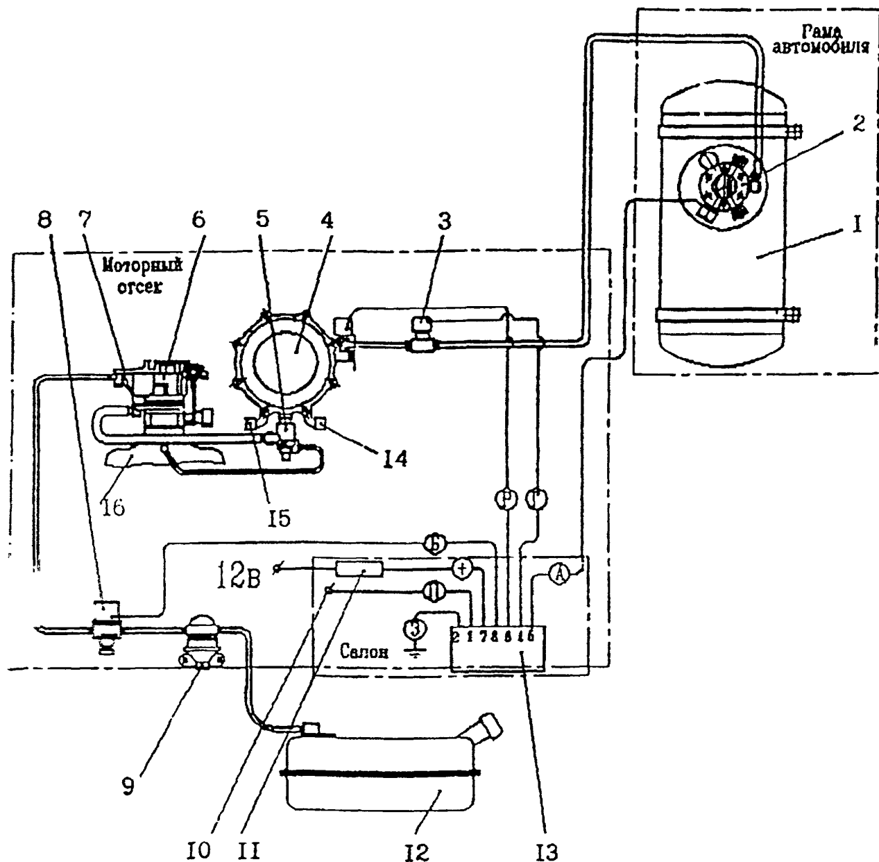
Рис. 3.3. Схема принципиальная газобаллонной установки АО «ЭКОРТ» для грузовых автомобилей:
