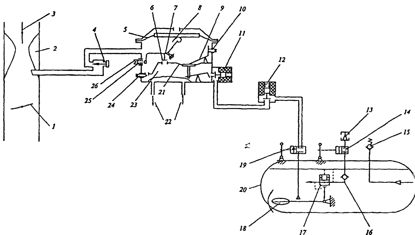
Рис. 3.1. Принципиальная схема основных элементов ГБО для ГСН:
