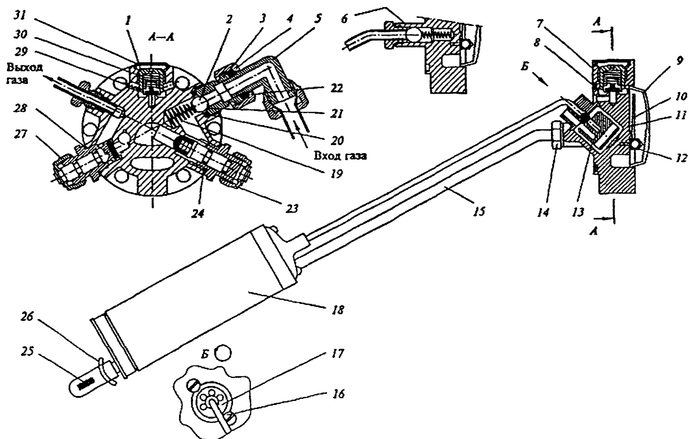
Рис. 3.8. Мультиклапан Новоградского завода газовой аппаратуры:
