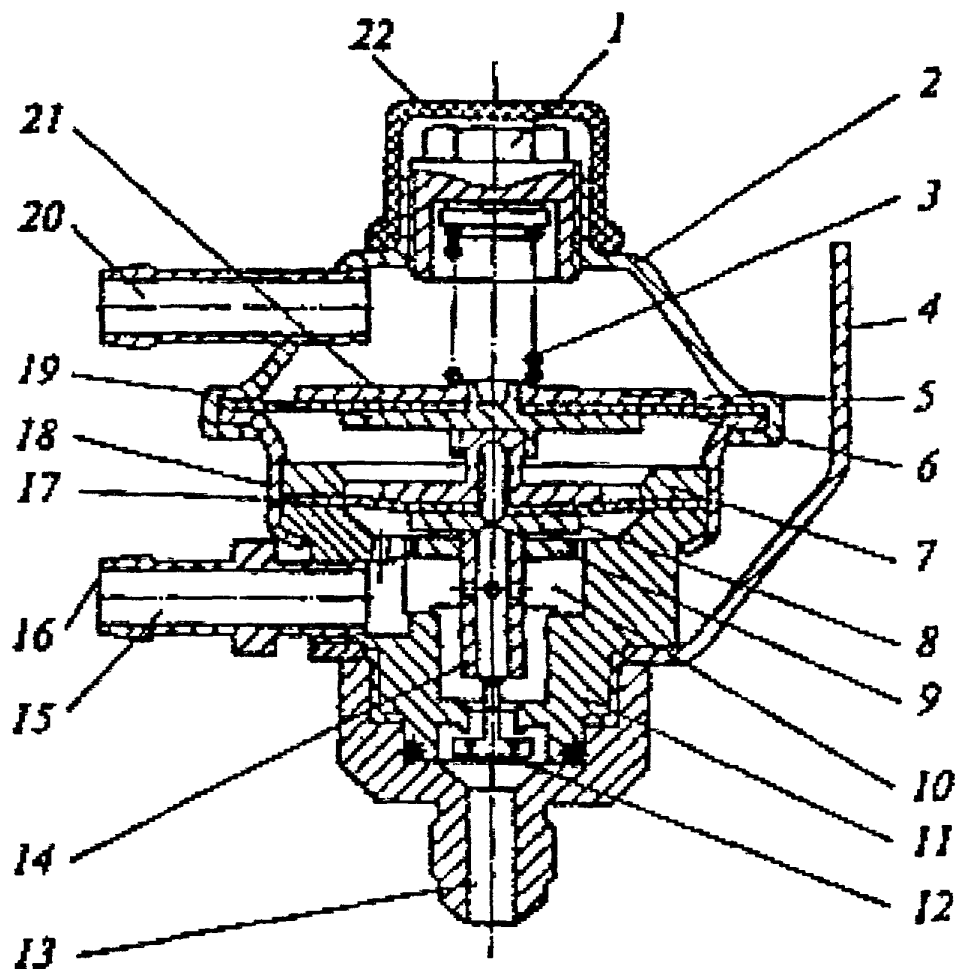
Рис. 3.11. Редуктор дифференциальный:
