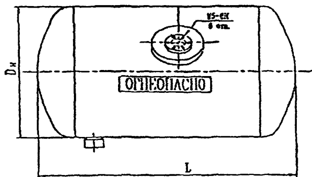
Рис. 3.7. Баллоны автомобильные газовые:
