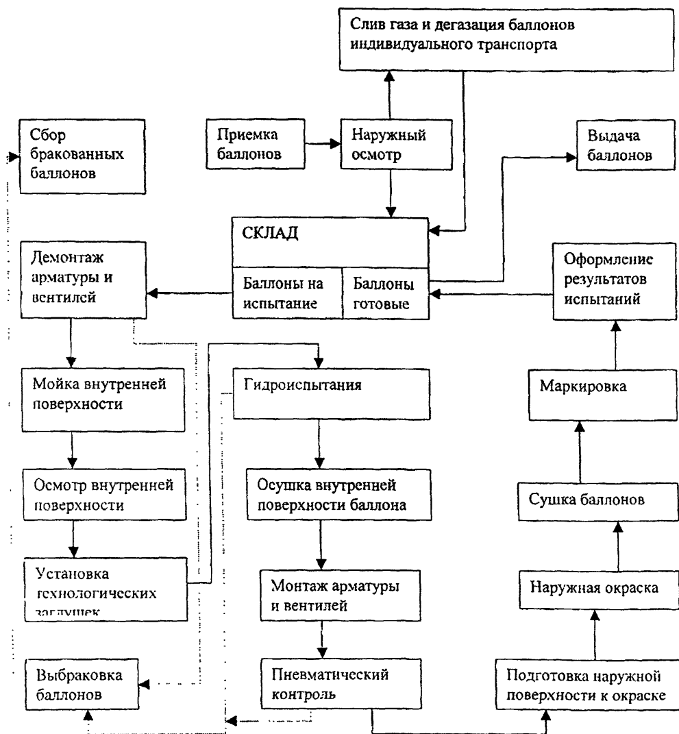
Рис. 9.1. Схема технологического процесса освидетельствования баллонов для ГСН
