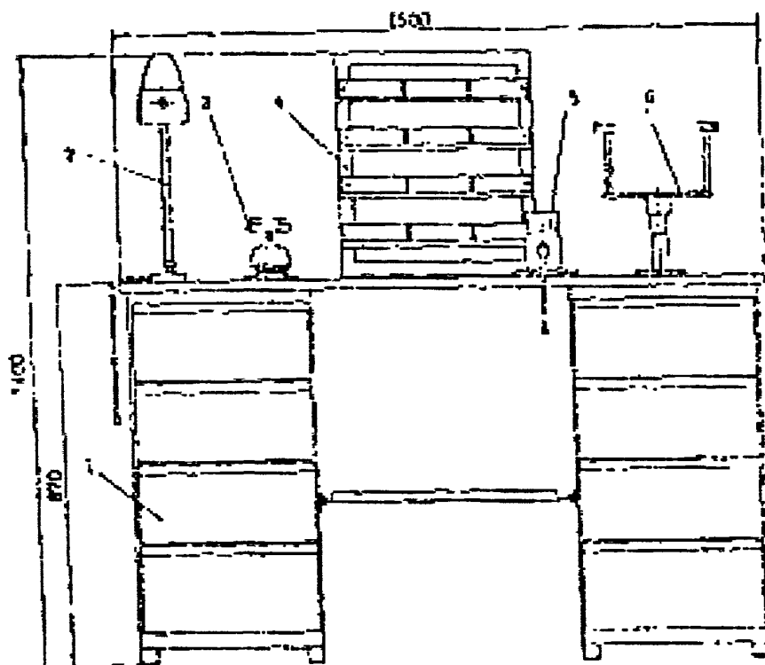
Рис. 6.3. Пост Р-991 для текущего ремонта газовой аппаратуры:
