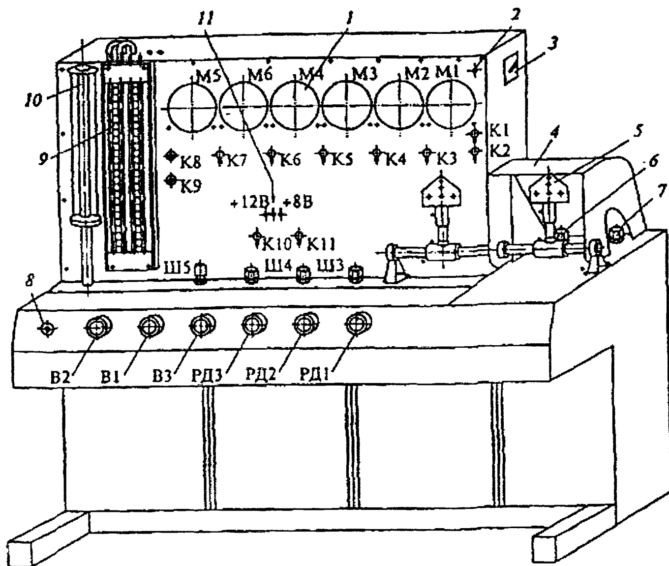
Рис. 6.4. Стенд ИС-001:
