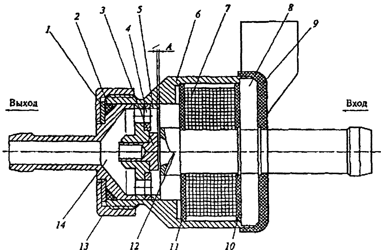
Рис. 3.12. Инжектор газовый:
