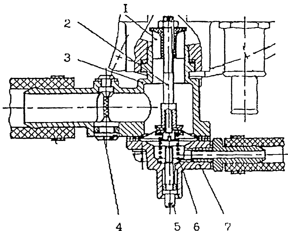
Рис. 4.1. Экономайзер:
