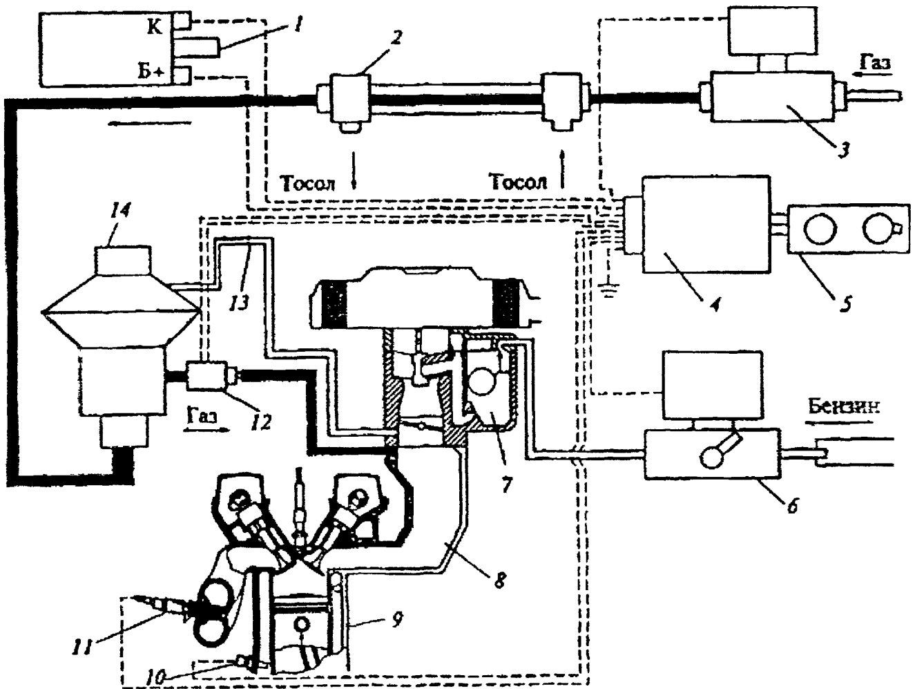
Рис. 3.10. Схема инжекторной системы дозирования газового топлива:
