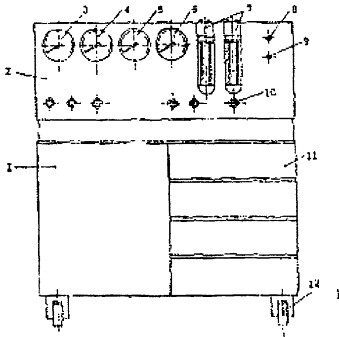
Рис. 6.1. Передвижная установка К-277 для проверки аппаратуры автомобилей:
