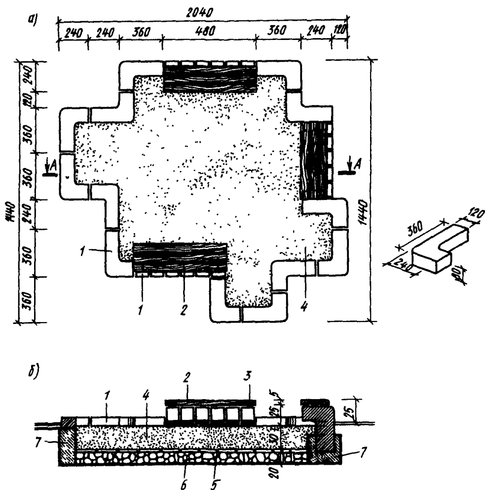
Рис. 20. Песочный дворик (опыт НРБ) а - план; б - разрез I - бетонный модульный элемент; 2 - деревянный элемент; 3 - планка; 4 - песок (30 см); 5 - кирпич; 6 - песок, глина; 7 - бетон
