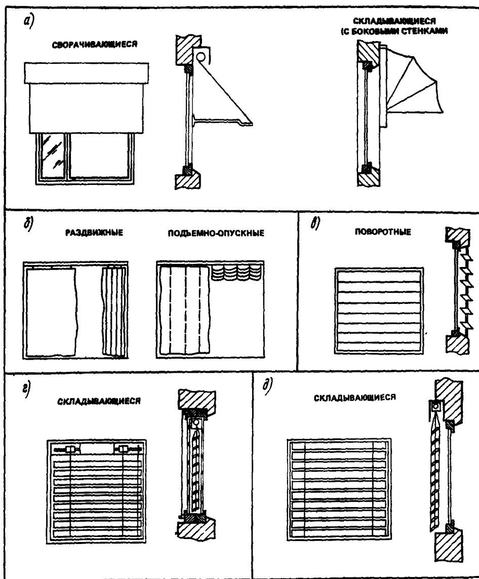
Рис. 33. Схемы СЗУ
