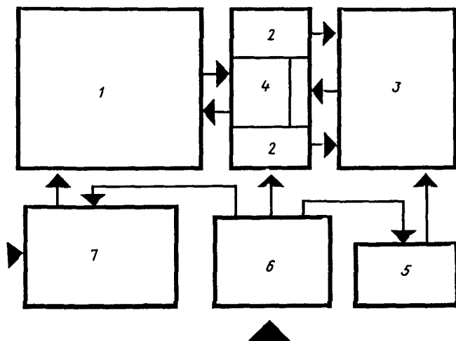
Рис. 46. Схема функциональной взаимосвязи помещений бассейна 1 - бассейн; 2 - раздевальня; 3 - зал для подготовительных занятий; 4 - душ; 5 - методический кабинет, класс; 6 - вес- тибюль; 7 - административно-бытовые помещения
