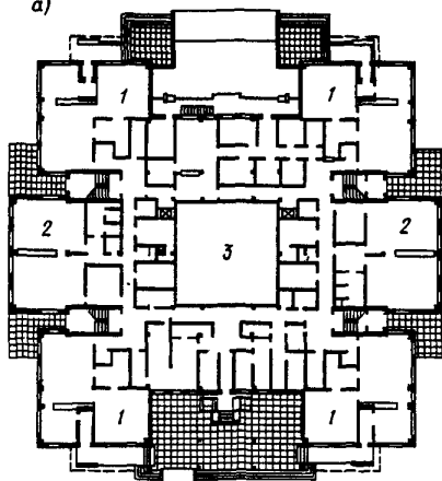
Рис.2. Схема организации комплексов дошкольных учреждений в одном здании (ЦНИИЭП учебных зданий )
