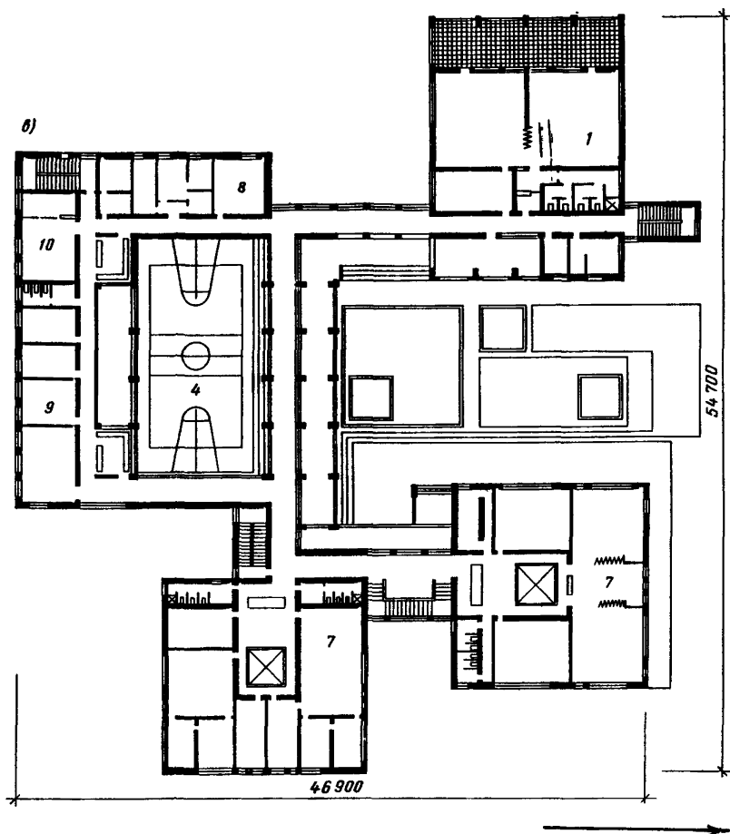
Рис.5.Кооперированное здание яслей-сада на 95 мест с начальной школой на 40 учащихся (Эстонская ССР, пос. Янеда) а - фасад; б - план 1-го этажа; в - план 2-го этажа 1 - вестибюль; 2 - физкультурный зал; 3 - столовая; 4 - групповые ячейки яслей-сада; 5 - пищеблок; 6 - медицинские помещения; 7 - административные помещения; 8 - классные помещения; 9 - рекреация; 10 - второй свет физкультурного зала
