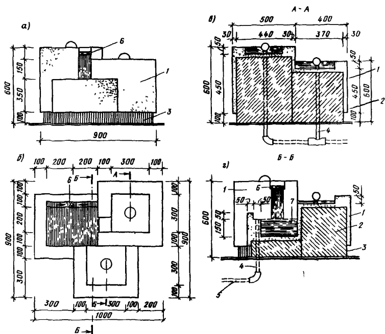
Рис. 24. Фонтанчики для игр с водой (опыт НРБ)
