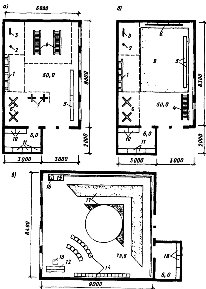
Рис. 45. Расстановка оборудования в залах специализированных детских учреждений
