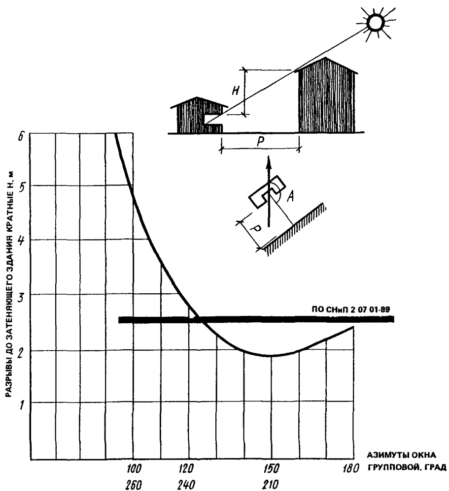
Рис. 9. График для определения величины разрыва между дошкольным учреждением и затеняющим объектом на равнине (ЦНТТЭП учебных зданий)
