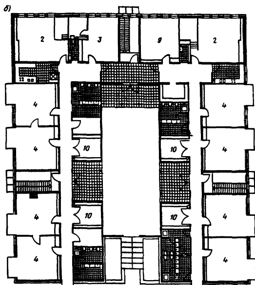
Рис. 26. Компактная схема объемно-планировочного решения здания детского сада на 170 мест (ФРГ)
