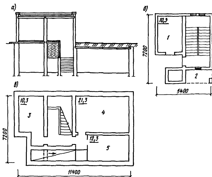
Рис. 25. Пример решения погреба-овощехранилища
