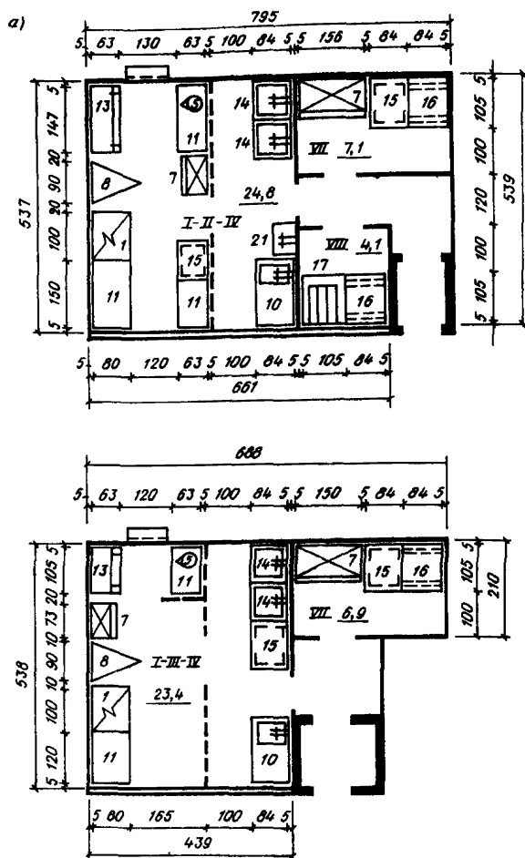
Рис. 49. Примеры планировок пищеблоков вместимостью а - до 50 мест; б - свыше 150 и до 250 мест; в - свыше 250 и до 350 мест;
