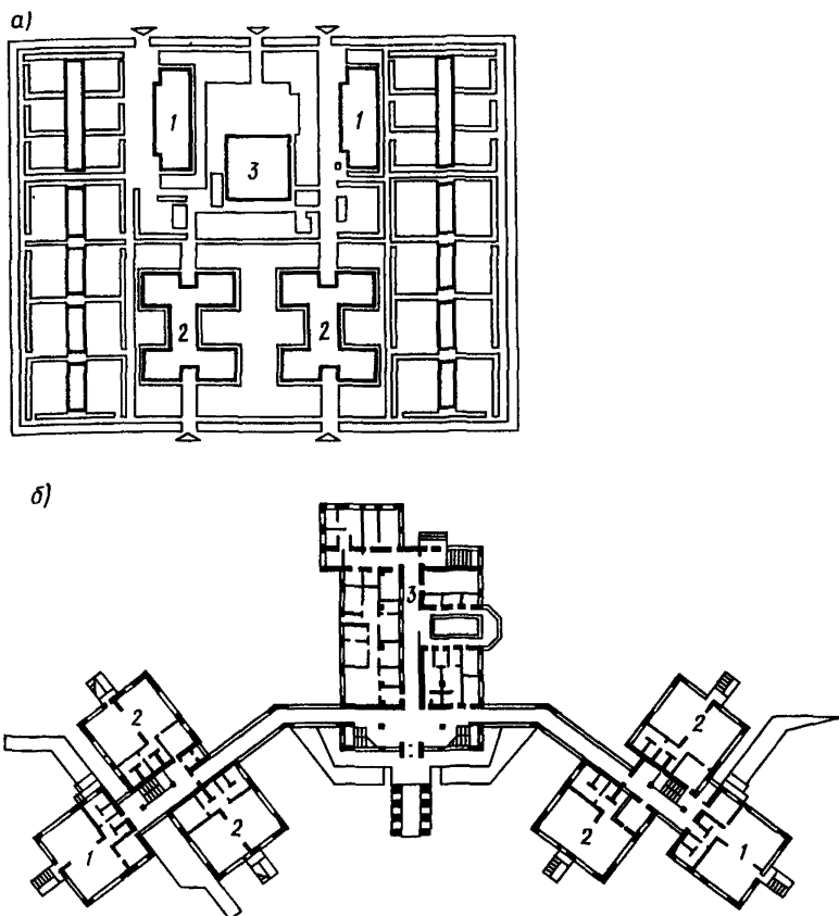
Рис. 1. Схема организации комплексов дошкольных учреждений (ЦНИИЭП учебных зданий) а - в виде отдельно стоящих зданий; б - в виде корпусов, соединенных переходом 1 - корпус ясельных групп; 2 - корпус групп детского сада; 3 - служебно-бытовое здание
