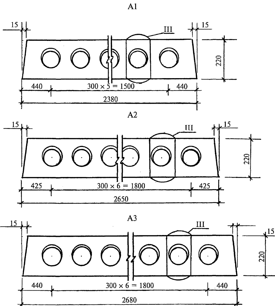
Узел III см. документ 1.041.1-5.0.1-5
