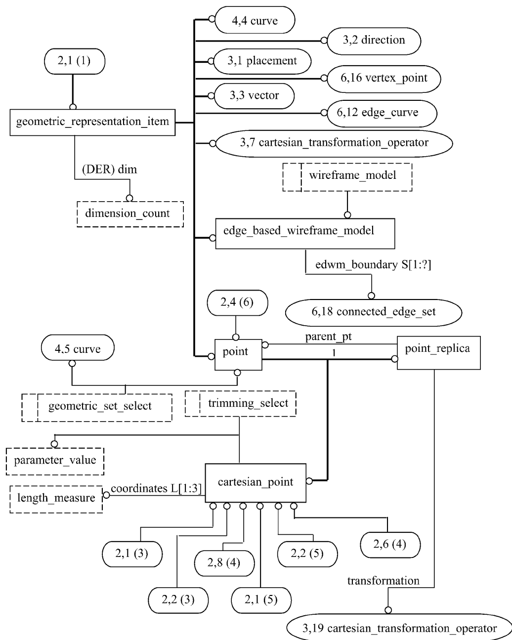
Рисунок С.2 — aic_edge_based_wireframe — EXPRESS-G диаграмма 2 из 6
