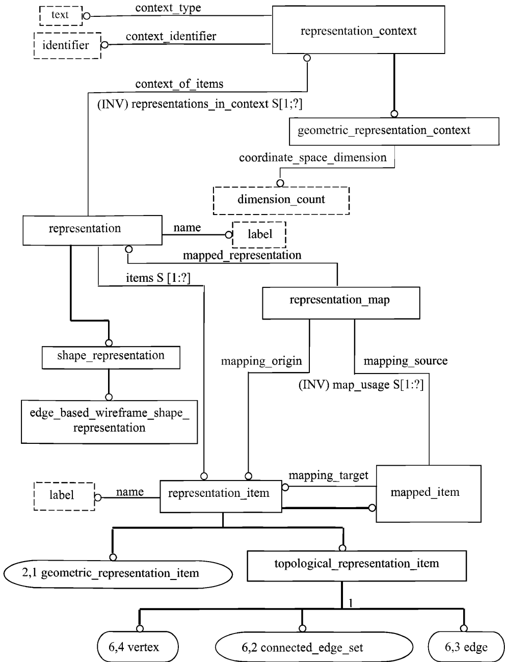
Рисунок С.1 — aic_edge_based_wireframe — EXPRESS-G диаграмма 1 из 6
