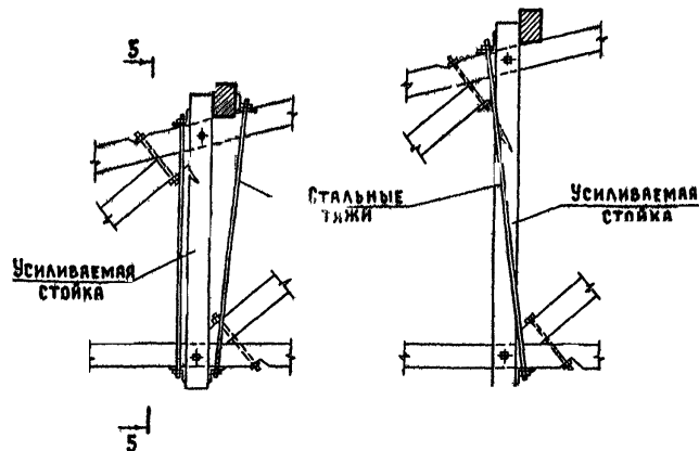
Усиление разорванной деревянной стойки стальными тяжами
