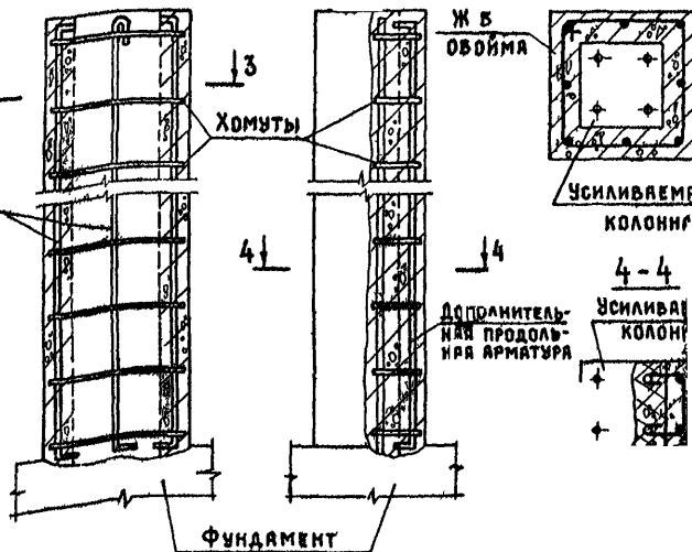
УСИЛЯЕМАЯ КОЛОННА
