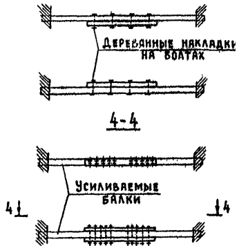
Усиление балок в середине пролета
