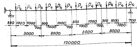
Элемент B2 (для расчета на местный изгиб).
