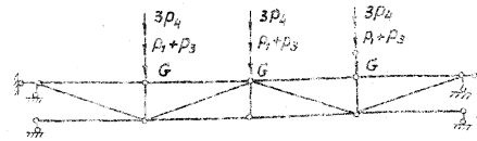
Элемент B2 (для расчета на местный изгиб).
