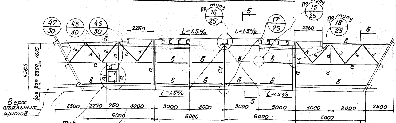
Фонарь шириной 12м; Нс=3500мм.
