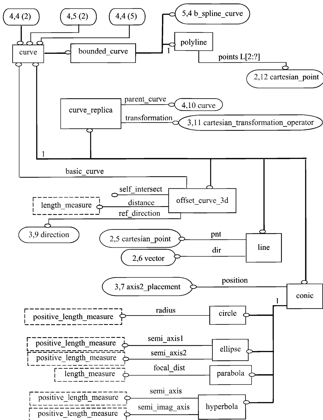
Рисунок С.4 — aic_shell_based_wireframe — EXPRESS-G диаграмма 4 из 6
