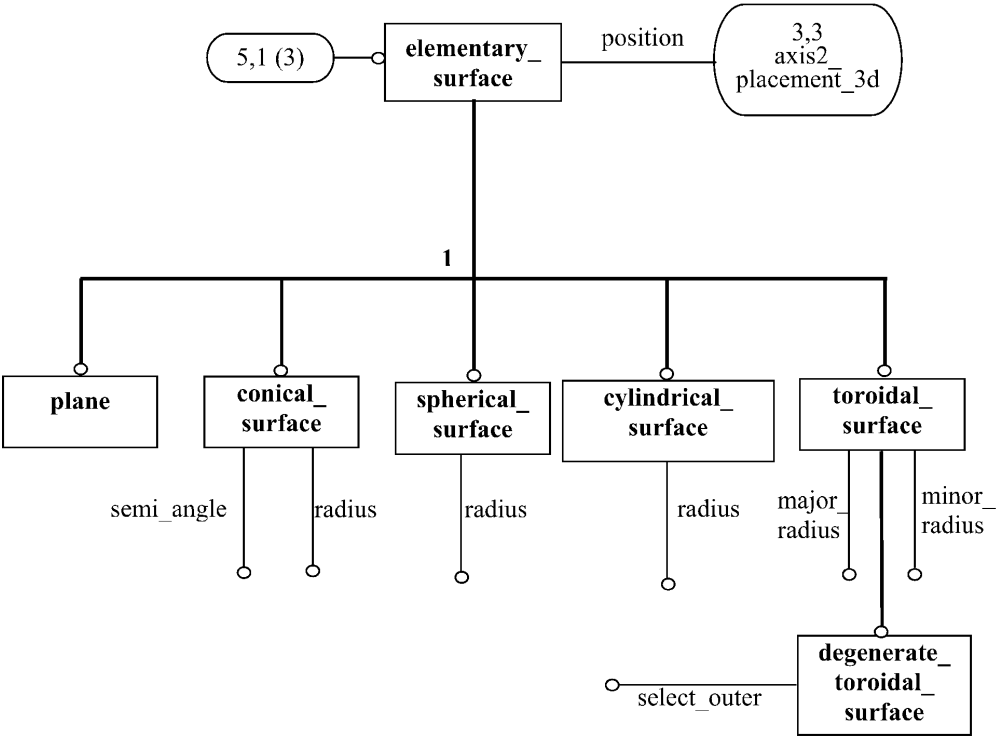
Рисунок D.5 — aic_topologically_bounded_surface — EXPRESS-G диаграмма 5 из 8
