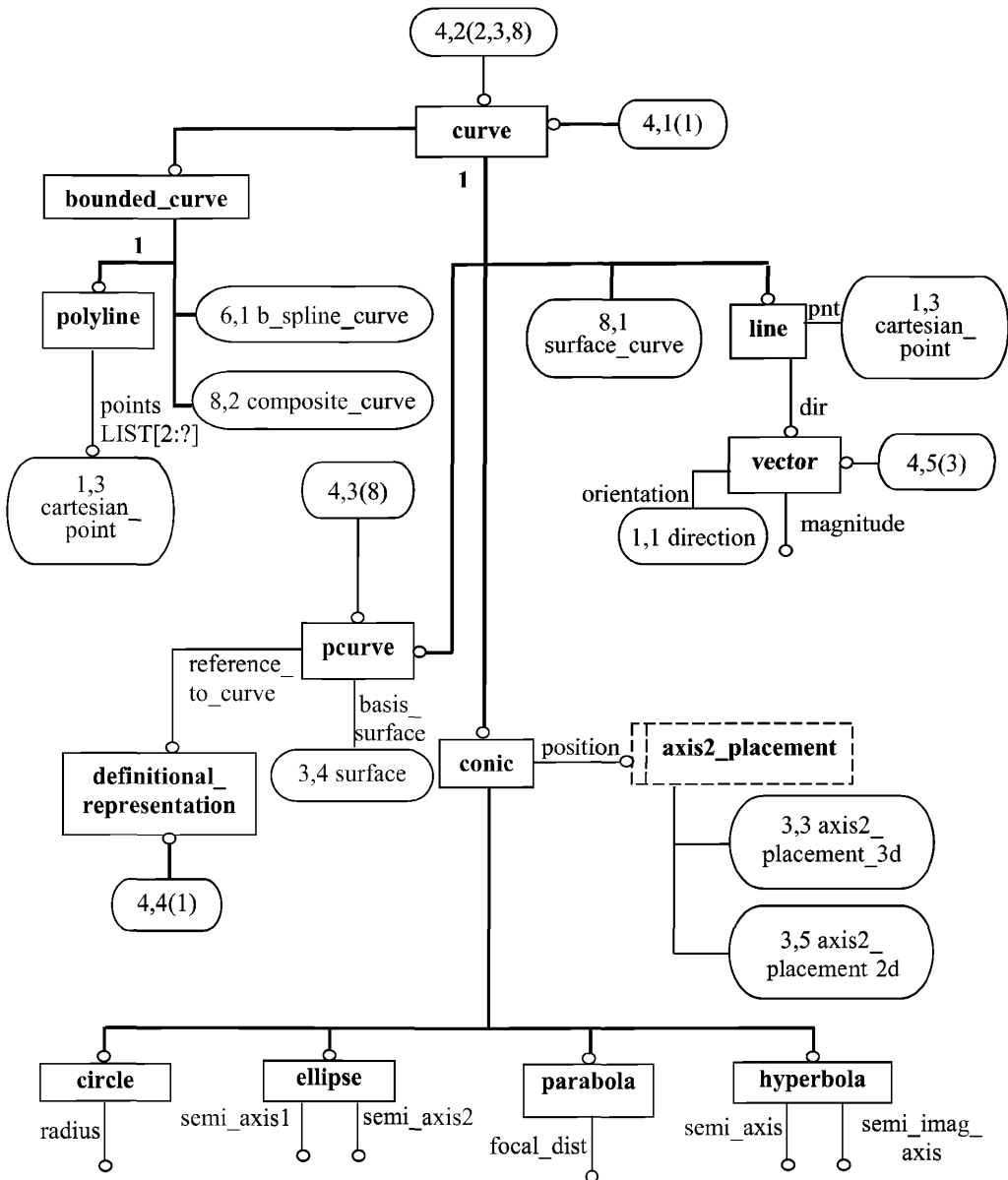
Рисунок D.4 — aic_topologically_bounded_surface — EXPRESS-G диаграмма 4 из 8
