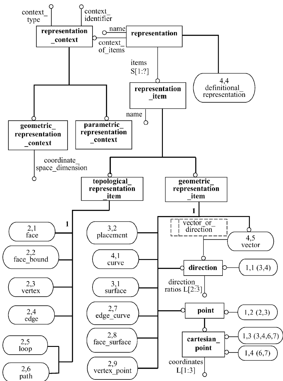
Рисунок D.1 — aic_topologically_bounded_surface — EXPRESS-G диаграмма 1 из 8
