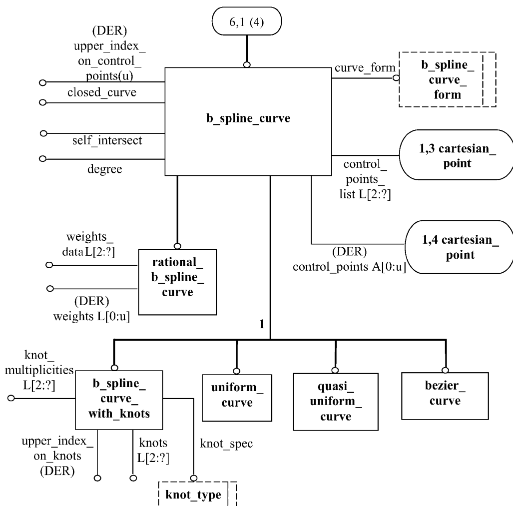
Рисунок D.6 — aic_topologically_bounded_surface — EXPRESS-G диаграмма 6 из 8
