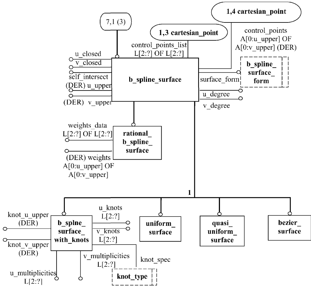
Рисунок D.7 — aic_topologically_bounded_surface — EXPRESS-G диаграмма 7 из 8
