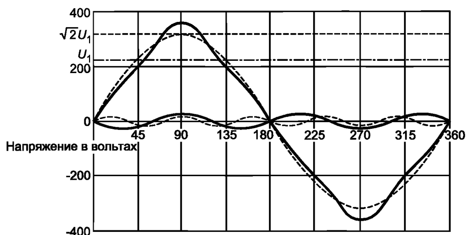
Рисунок 6 — Форма испытательного сигнала при испытаниях «Треугольные импульсы»
