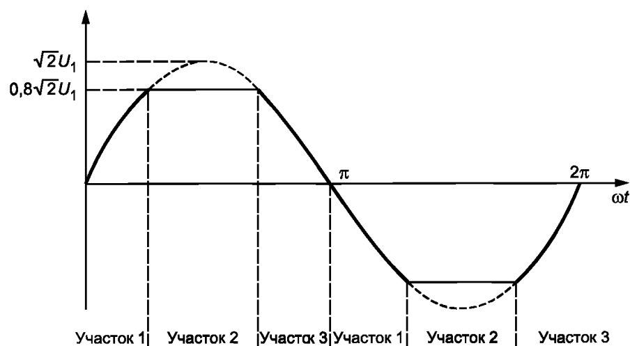
Рисунок 5 — Форма испытательного сигнала при испытаниях «Ограниченная синусоида»
