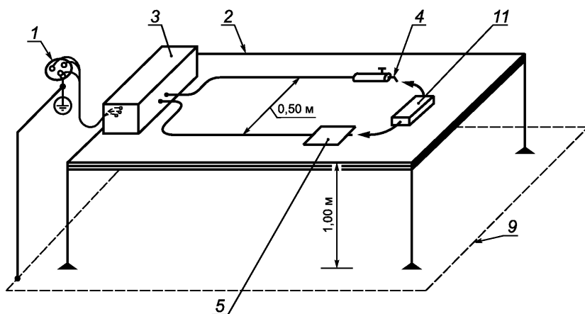
Рисунок 105 — Измерение ВЫХОДНОЙ МОЩНОСТИ. Монопольный выход (пункт 50)
