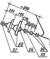
Анкеровка стальных проводов
