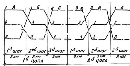
Схема транспозиции ВЛВ проводов
