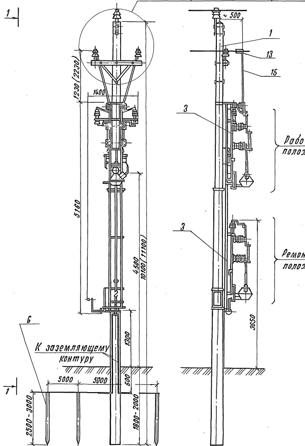
1-1 Оснстка промежуточной опоры
