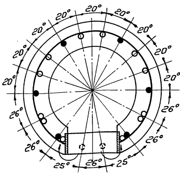
СНЦс - 5,1 - 11,5
