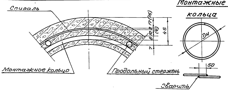
Деталь поперечного сечения стойки.
