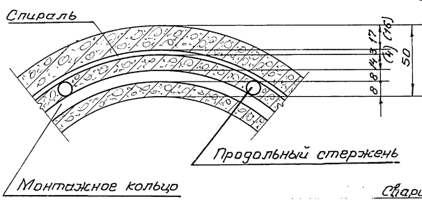
Деталь поперечного сечения стойки.
