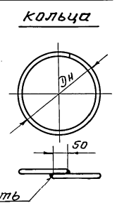
Монтажные кольца
