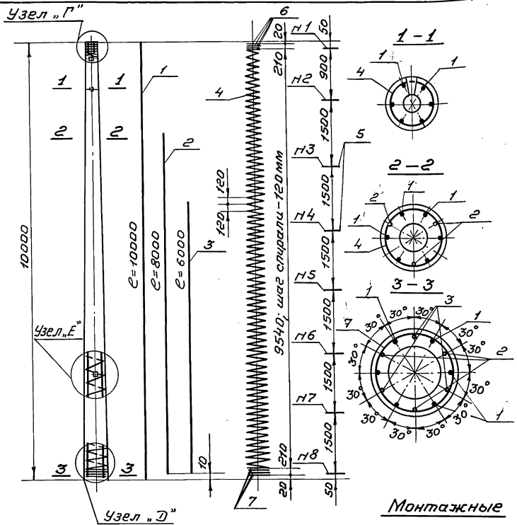
Деталь поперечного сечения стойки.
