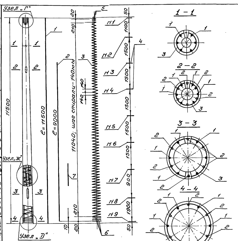
Деталь поперечного сечения стойки.
