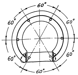
СНЦс - 5,1 - 11,5
