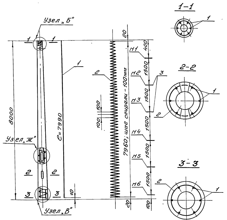
Деталь поперечного сечения стойки.
