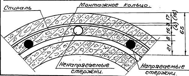
Деталь поперечного сечения стойки.
