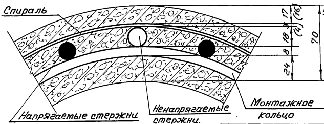
Деталь поперечного сечения стойки.
