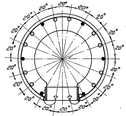
СНЦс - 10 - 12
