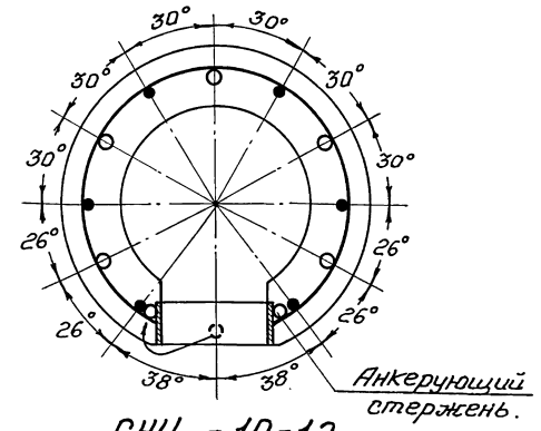
СНЦс - 10 - 12
