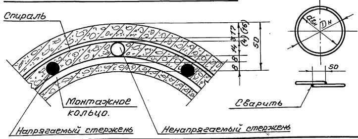
Деталь поперечного сечения стойки.
