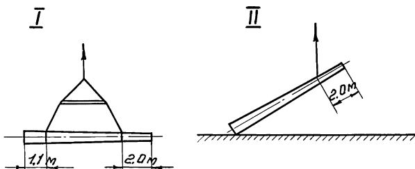
Схемы подъема стойки.
