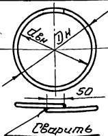
Монтажные кольца и хомуты.
