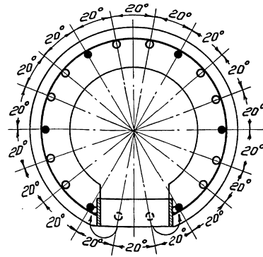
СНЦс - 7,7 - 12
