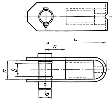
Втулка ВТО
