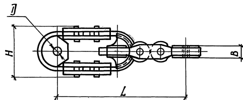
Изолятор ЦИ-1
