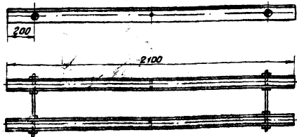
Траверса ВЛ-10кВ; Т-3 (для концевой и ответвительной опоры)
