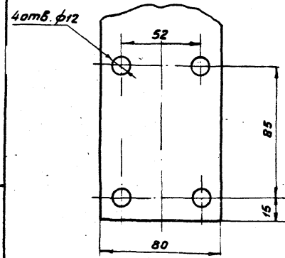
Вид по А
