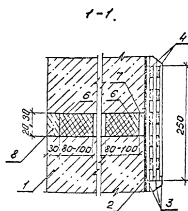
б) стенки
