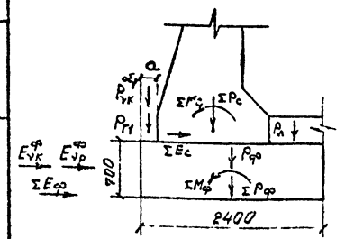
Схема нагрузок
