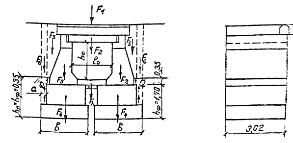
Расчетные схемы оголовочных секций для глубины промерзания d_{zh}=2,0 м
