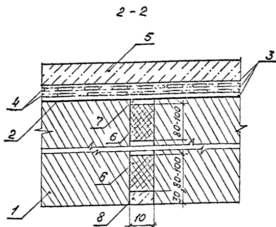
а) ригеля
