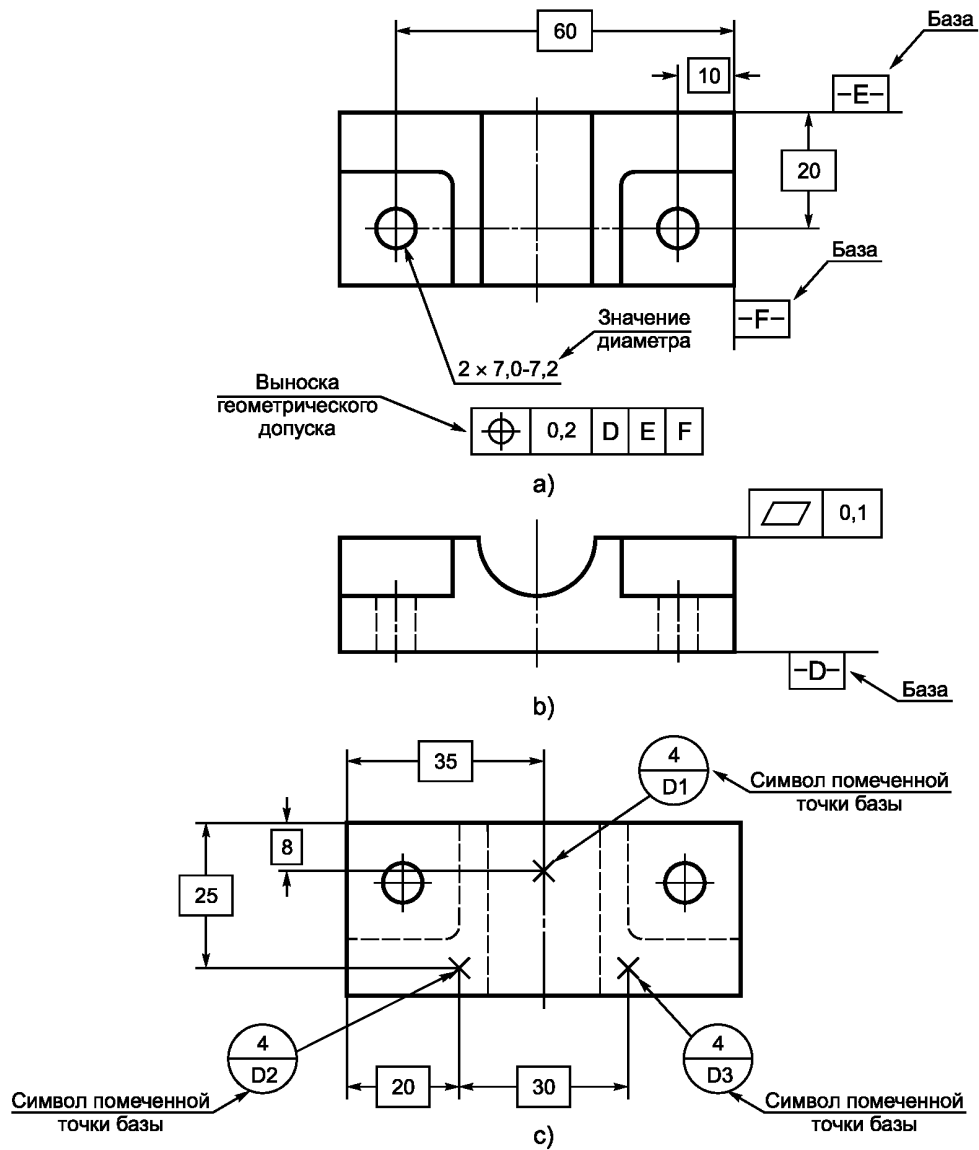
Рисунок 3 — Чертежные выноски
