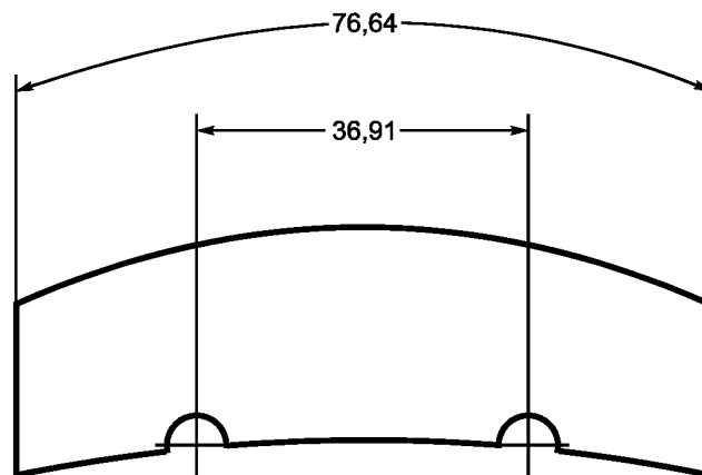
Рисунок 2 — Размер дуги
