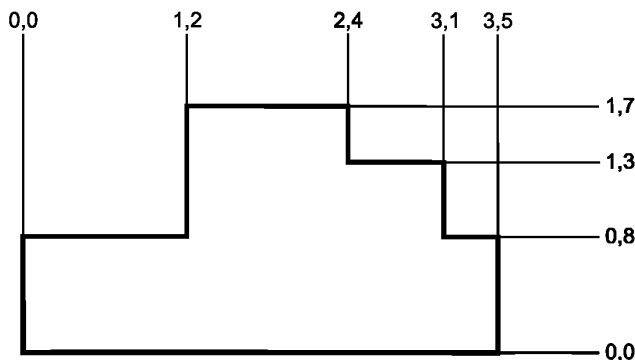
Рисунок 9 — Ординатный размер
