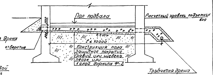
Разрез 2-2
