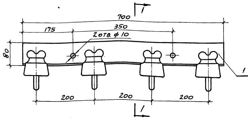
СКОБА М 1:1
