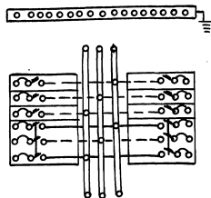
Типовая схема щитков серии СУ9400
