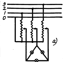
Схема включения темнителя света ТС-5 в сеть 220/127 вольт
