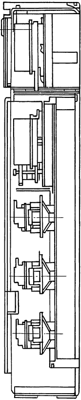
РАЗРЕЗ I-I
