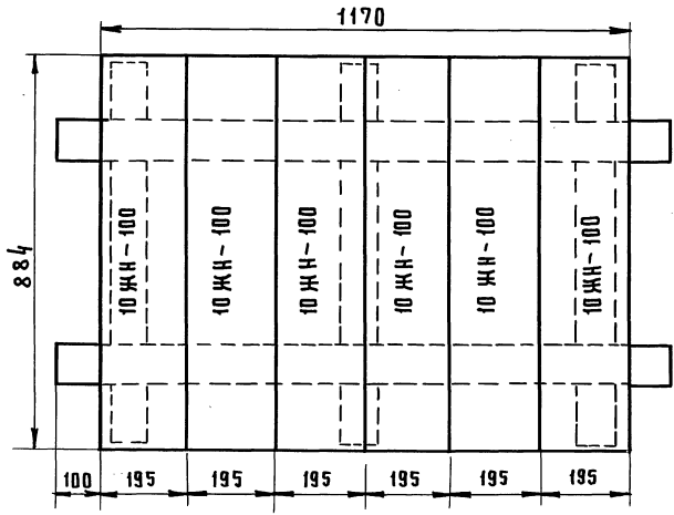
Расположение аккумуляторных батарей на стеллаже в плане (м:10)
