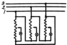
Схема включения темнителя света ТС-6 в сеть 220В
