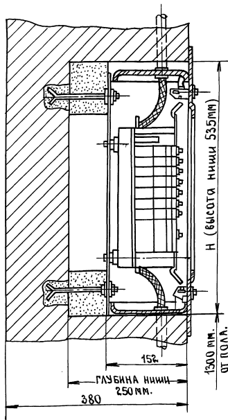
Типовая схема щитков серии СУ9400
