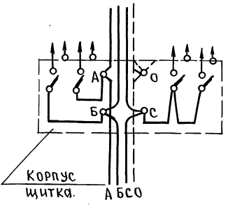
Монтажная схема.
