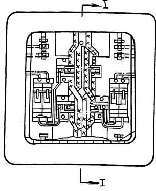
Вид со снятой дверцей
