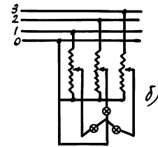
Схема включения темнителя света ТС-5 в сеть 220/127 вольт
