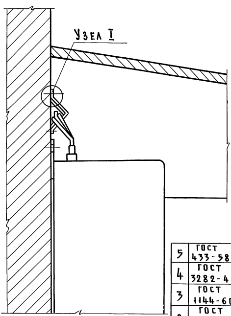
РАЗРЕЗ 1-1
