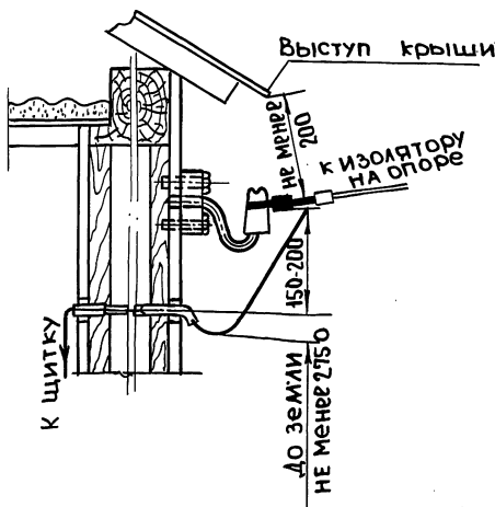
Ввод в щитовое и глино-плетневое здание нормальной высоты.
