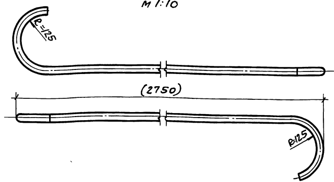
ТРУБА М 1:10
