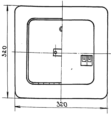
Этажный щиток типа ЩЭ-7
