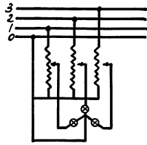
Схема включения темнителя света ТС-6 в сеть 380/220В
