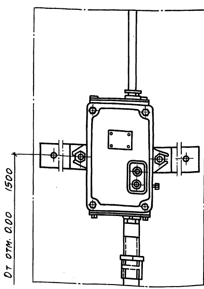
КРЕПЛЕНИЕ АВТОМАТА АП-50 В МЕТАЛЛИЧЕСКОМ КОЖУХЕ
