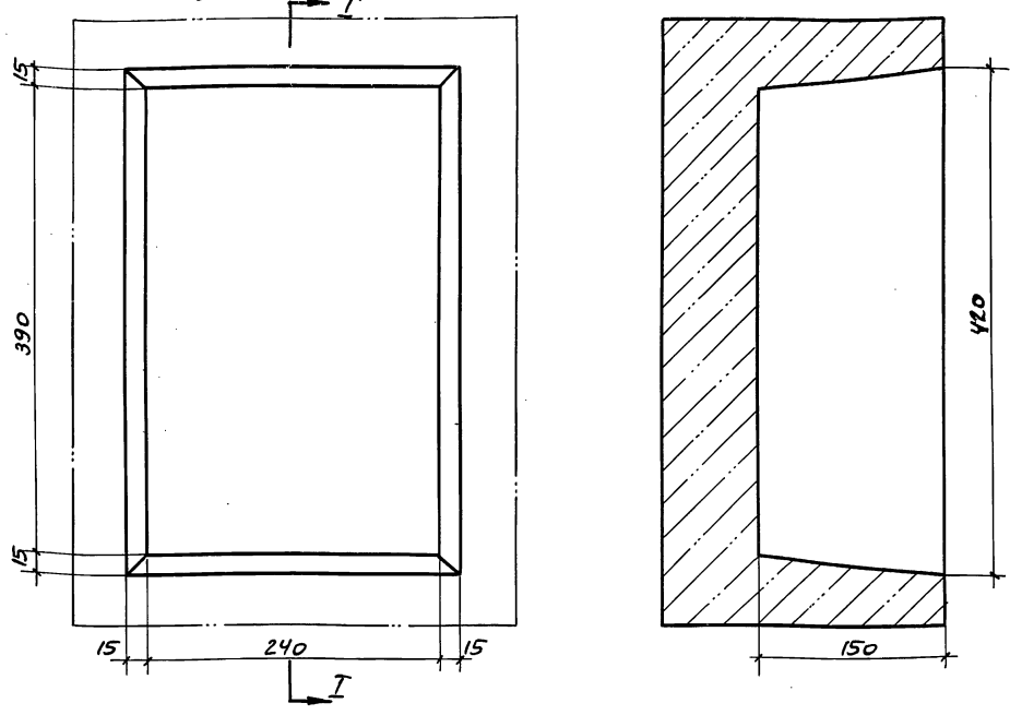
РАЗМЕРЫ НИШИ М 1:4 Вид СПЕРЕДИ РАЗРЕЗ I-I
