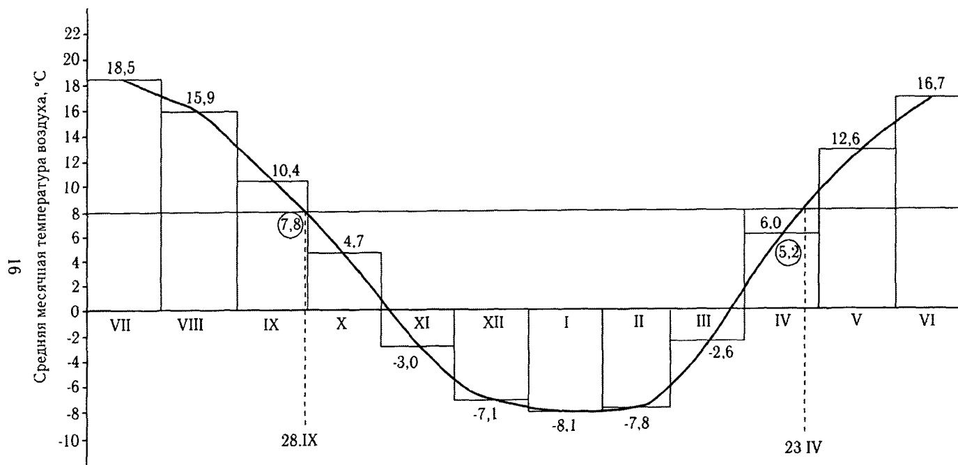
Рис. 1.3. График расчета продолжительности и средней температуры воздуха отопительного периода для г. Черусти
