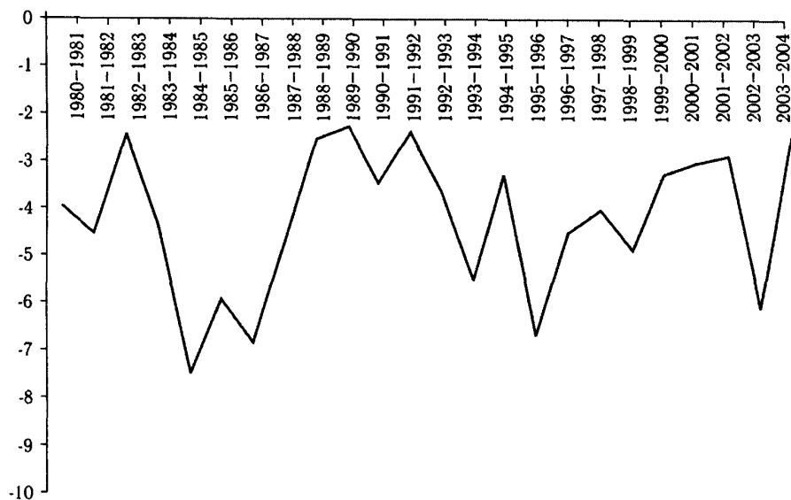
Рис. 5.6. Ход средних зимних месячных температур, г. Наро-Фоминск
