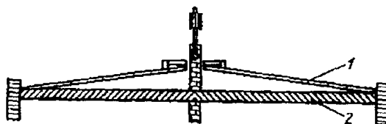
Рис. 29. Трипод со съемной визирной целью 1 — кривля; 2 — перекрытие (блика)
