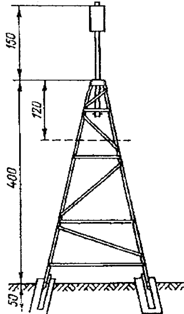
Рис. 26. Пирамида-штатив из уголковой стали ( 50 \times 50 \times 5 или 35 \times 35 \times 4 ) со съемной малофазной визирной целью с высотой до инструментального столешка от 1,5 до 0,4 м.
