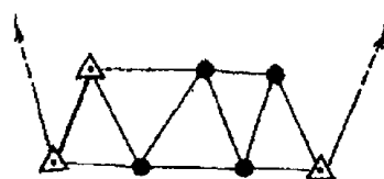
Рис. 23 Цепочка треугольников между стороной и пунктом
