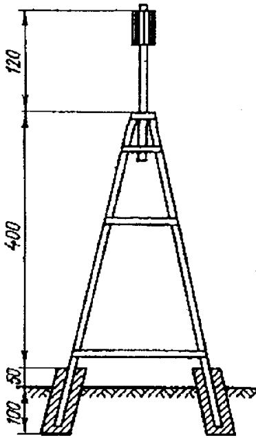
Рис. 25 Четырехгранная пирамида (из уголковой стали)
