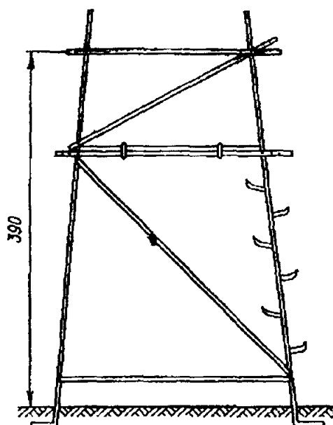
Рис. 27. Металлическая переносная площадка для наблюдения с пирамид-штативов. Изготавливается из уголкового стали ( 50 \times 50 \times 5 и 25 \times 35 \times 4 )
