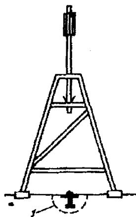
Рис. 30. Пирамидо-штатив со съёмной визирной делью 1 — марка триангуляционная
