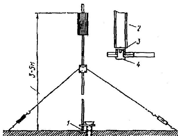
Рис. 31. Съёмная металлическая коробка с визирным цилиндром 1 — центр пункта; 2 — вежа, 3 — отверстие (центр пункта); 4 — болт
