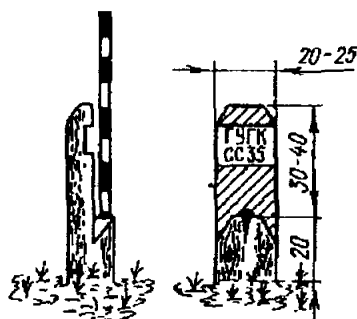
Рис. 44. Тип знака долговременного закрепления пунктов съёмочных сетей в залесенных районах
