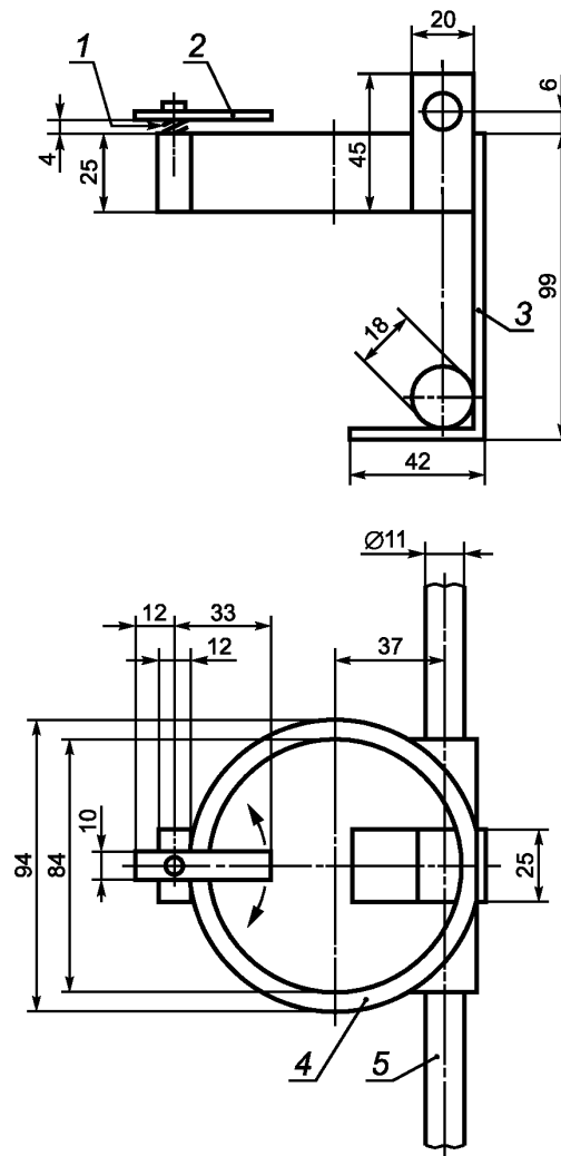
Рисунок 2 — Разливочное устройство
