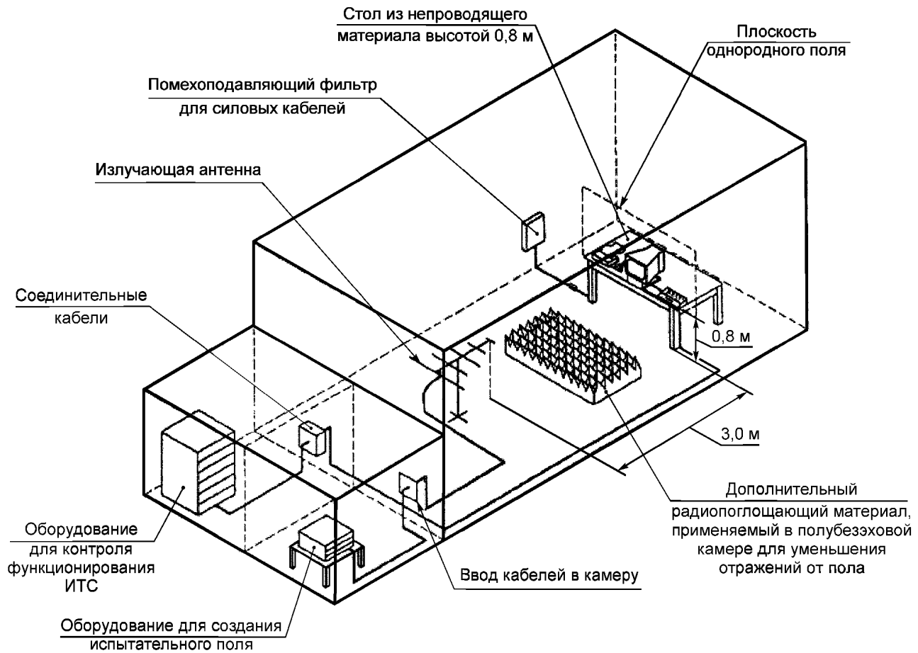
Рисунок 2 — Пример испытательной установки
