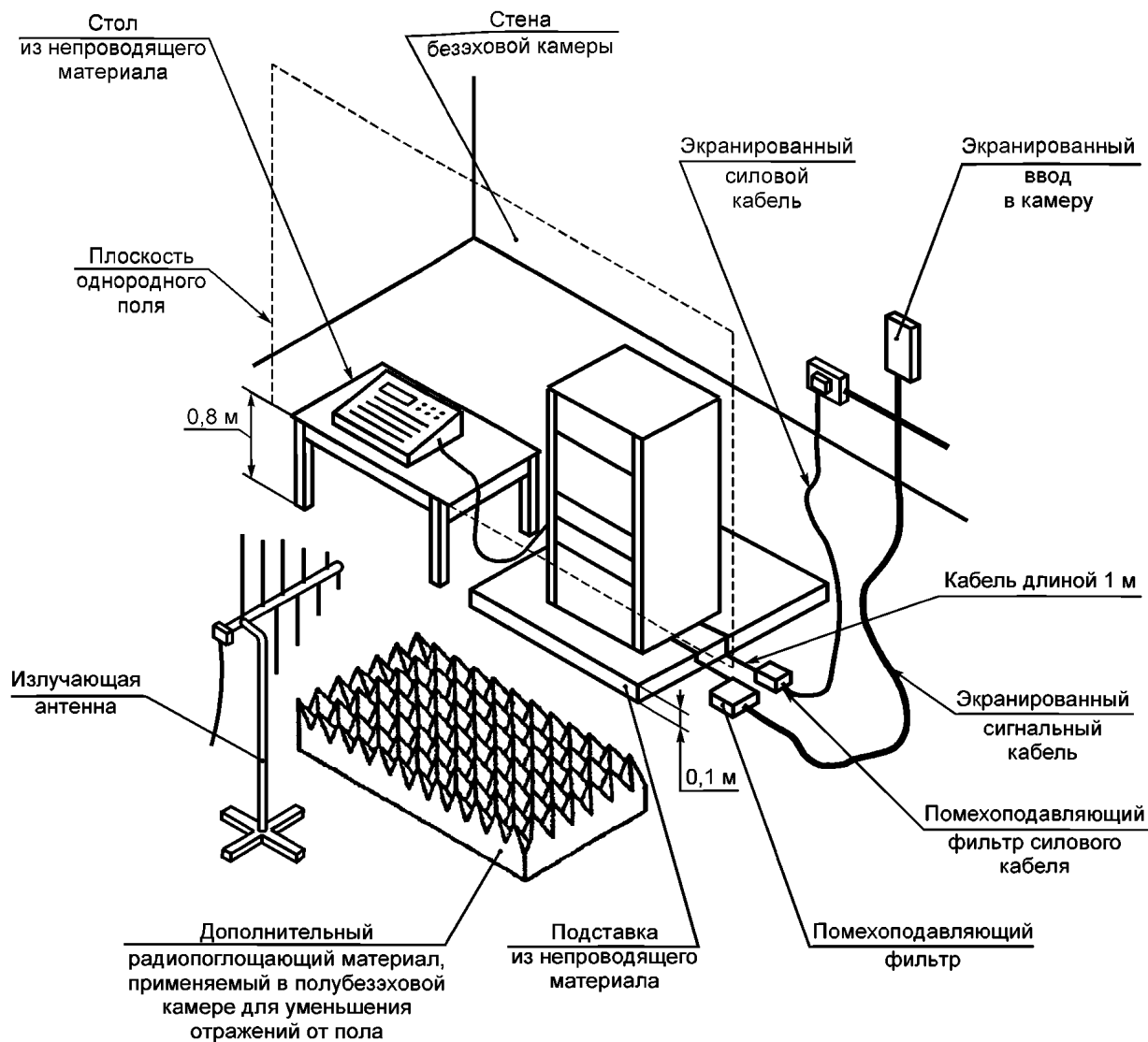
Рисунок 5 — Пример установки для испытаний напольных ТС
