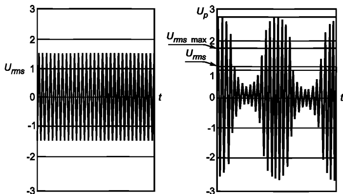
а) Немодулированный радиочастотный сигнал (пиковое значение напряжения U_p = 1,4 В, среднеквадратическое значение напряжения U_{rms} = 1 В);
