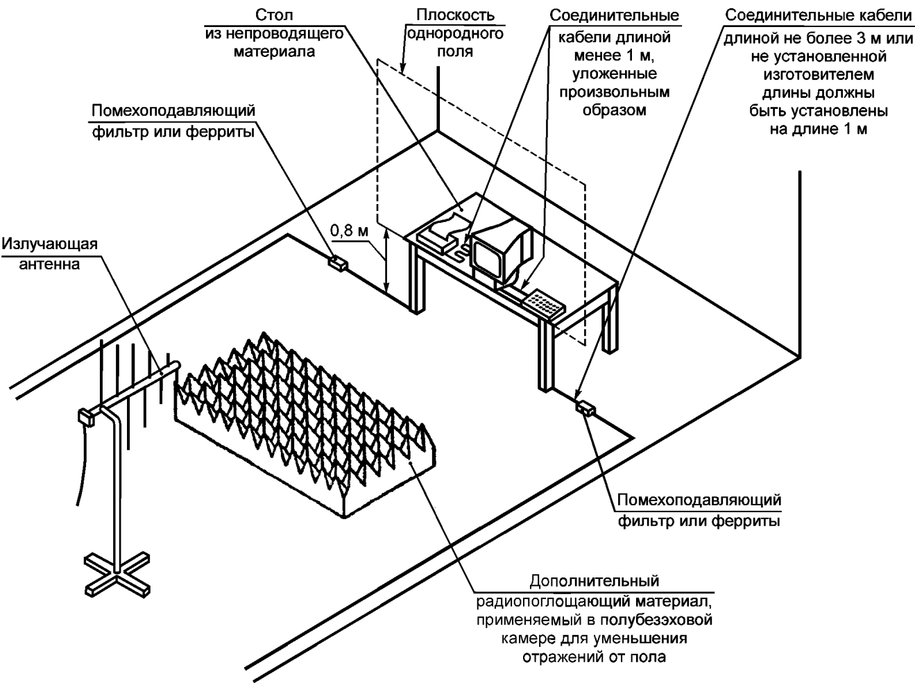
Рисунок 6 — Пример установки для испытаний настольных ТС
