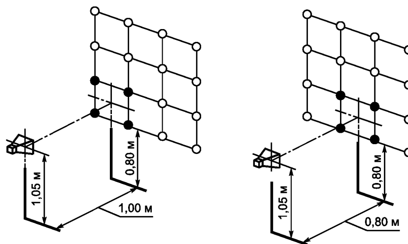
Рисунок И.2 — Пример последовательного облучения окон
