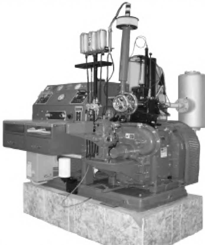
Рисунок 2 — Установка CFR F-5 для определения цетанового числа
