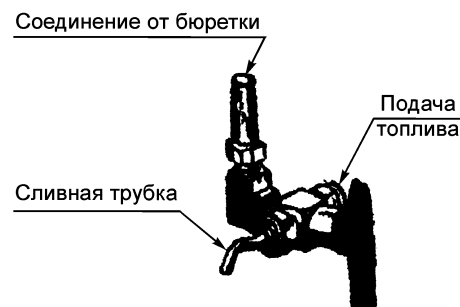
Рис. Б.2 — Типовой трехходовой кран для приготовления эталонных топлив
