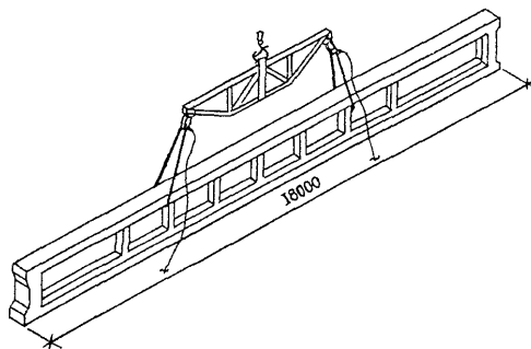
Траверса TP20-5
