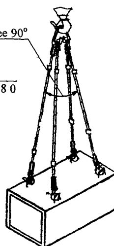
Строп 4СК1-20,0 Q = 20,0 тс при погрузке железобетонной секции P = 14,3 т
