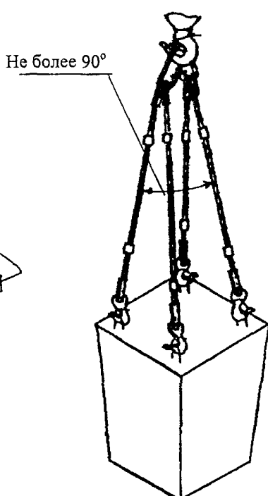
Строп 4СК1-3,2-4СК1-10,0 Q = 3,2-10,0 тс при разгрузке с транспорта подколонников P = 2,5 \text{ т}
