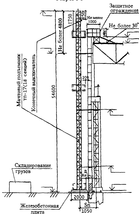
Разрез I-I
