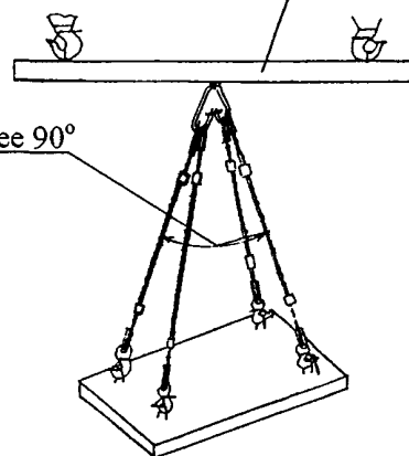
Траверса для монтажа двумя кранами
