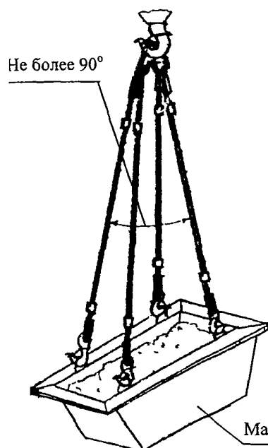
Строп 4СК1-3,2-4СК1-10,0 Q = 3,2-10,0 тс при подаче ящика с цементным раствором емкостью 0,28 \text{ м}^3 P = 0,65 \text{ т}
