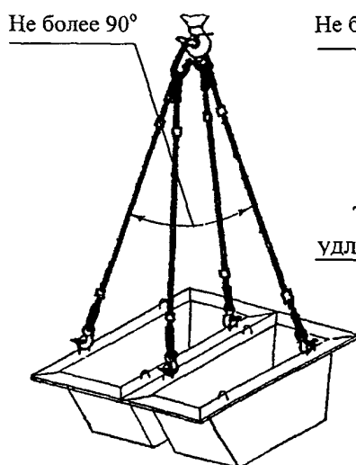
Строп 4СК1-3,2-4СК1-10,0 Q = 3,2-10,0 тс при подаче пустой тары P = 54 \times 2 = 108 \text{ кг}
