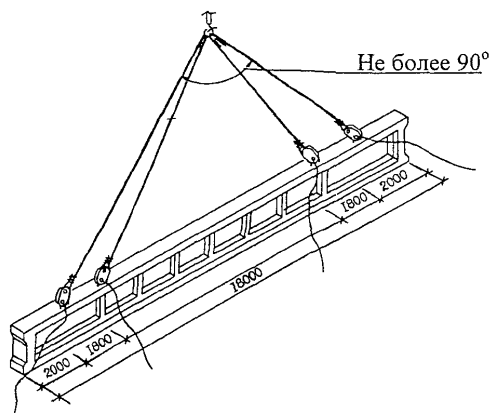
Строп 2СК-10,0
