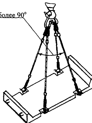
Строп 4СК1-3,2-10,0 Q = 3,2-10,0 тс при погрузке лоткового днища канала P = 0,74-2,85 т
