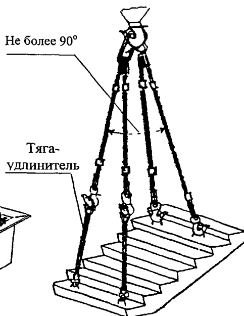
Строп 4СК1-3,2-4СК1-10,0 Q = 3,2-10,0 тс при монтаже лестничных маршей P = 0,865-1,98 \text{ т}
