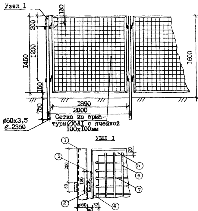
Рисунок 29 – Пример конструкции ограждения кранового пути высотой 1600 мм.
