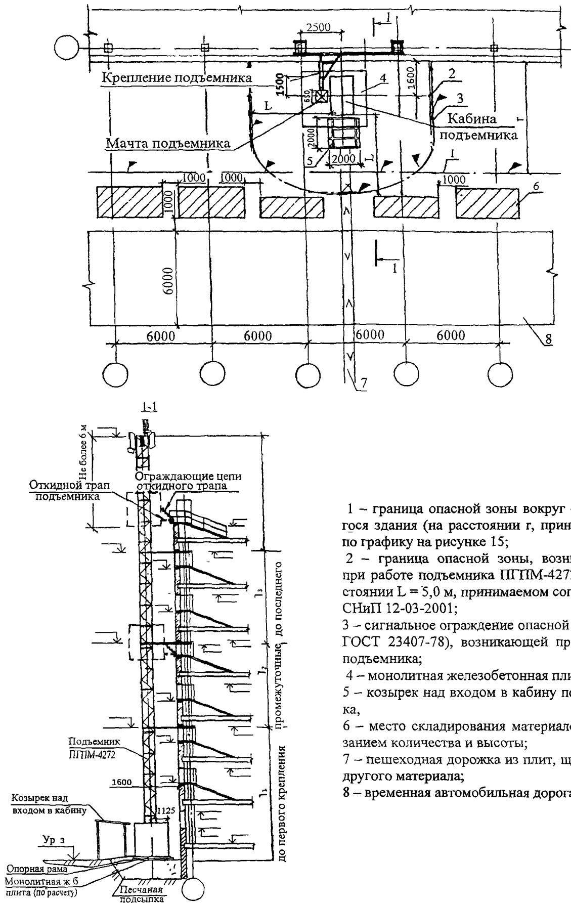
Рисунок 36 – Установка пассажирского подъемника ПГПМ-4272 у здания.
