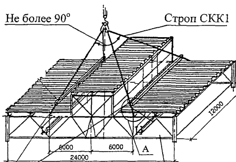
Блок покрытия пром зданий P_{\max}=22 \text{ т}
