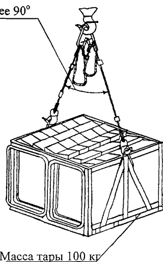
Строп 4СК1-5,0–4СК1-10,0 Q = 5,0–10,0 тс при разгрузке с автотранспорта кирпича в траверсном футляре Р = 1,7 т
