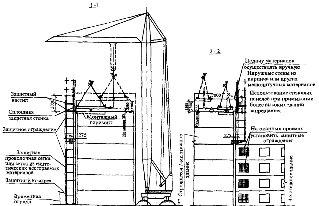
Рисунок 24 – Разрезы 1-1 и 2-2
