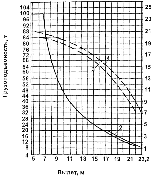
Стрела 21 м
