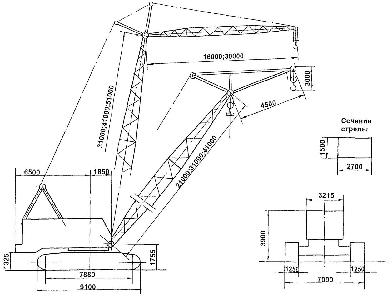
МКГ - 100
