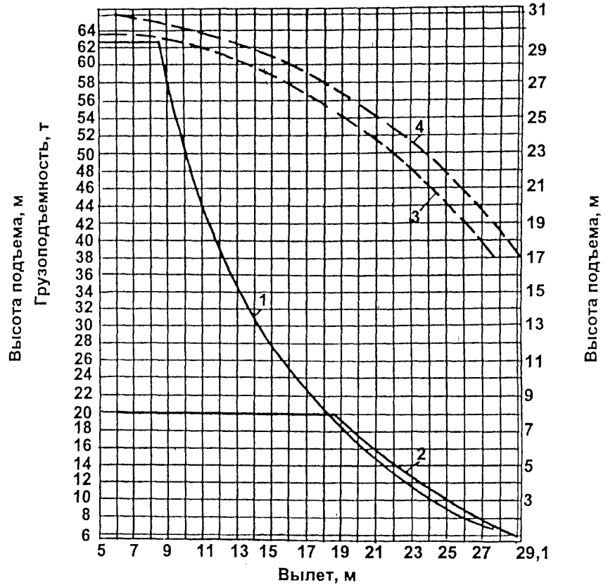
Стрела 31 м
