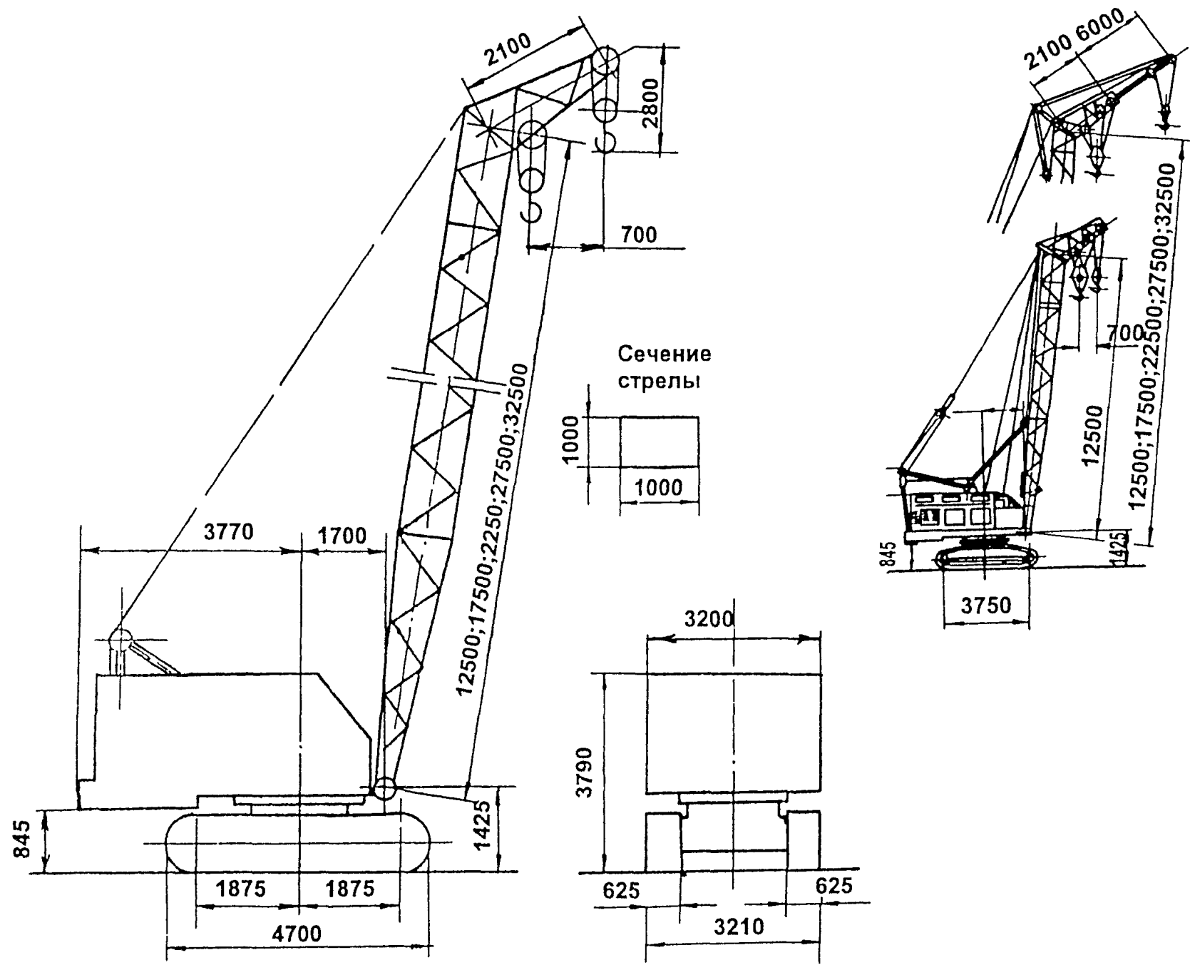
МКГ - 25
