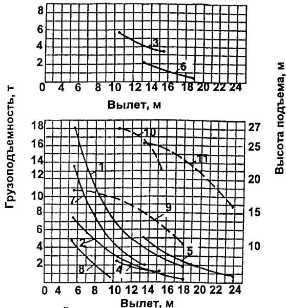
Стрела 20 м
