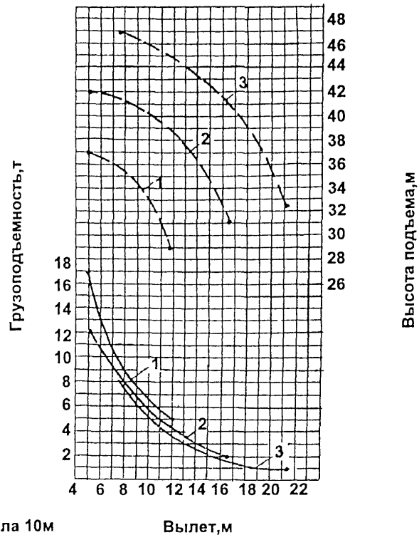
Башня 28,5 м
