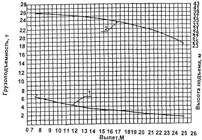
Башня 26 м
