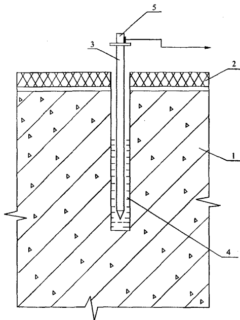
1 – монолитная конструкция; 2 – утеплитель; 3 – пенал из тонкостенной стальной трубы; 4 – индустриальное масло; 5 – термоматчик
