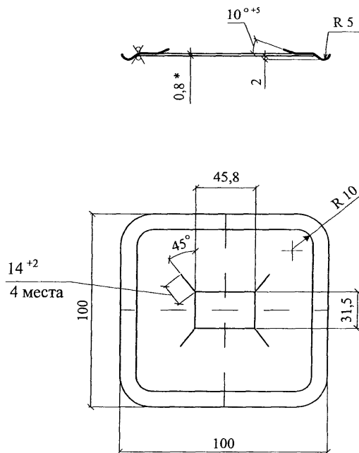
ПРИЖИМНАЯ ПЛАНКА
