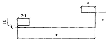
НАЩЕЛЬНИК Н2
