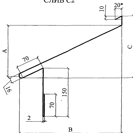
СЛИВ С2
