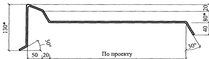
КОСТЫЛЬ К3
