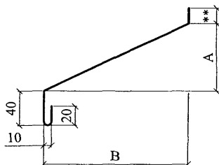
СЛИВ С3
