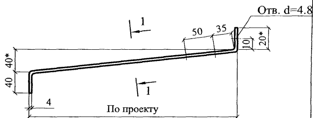
КОСТЫЛЬ К2
