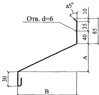
СЛИВ С3
