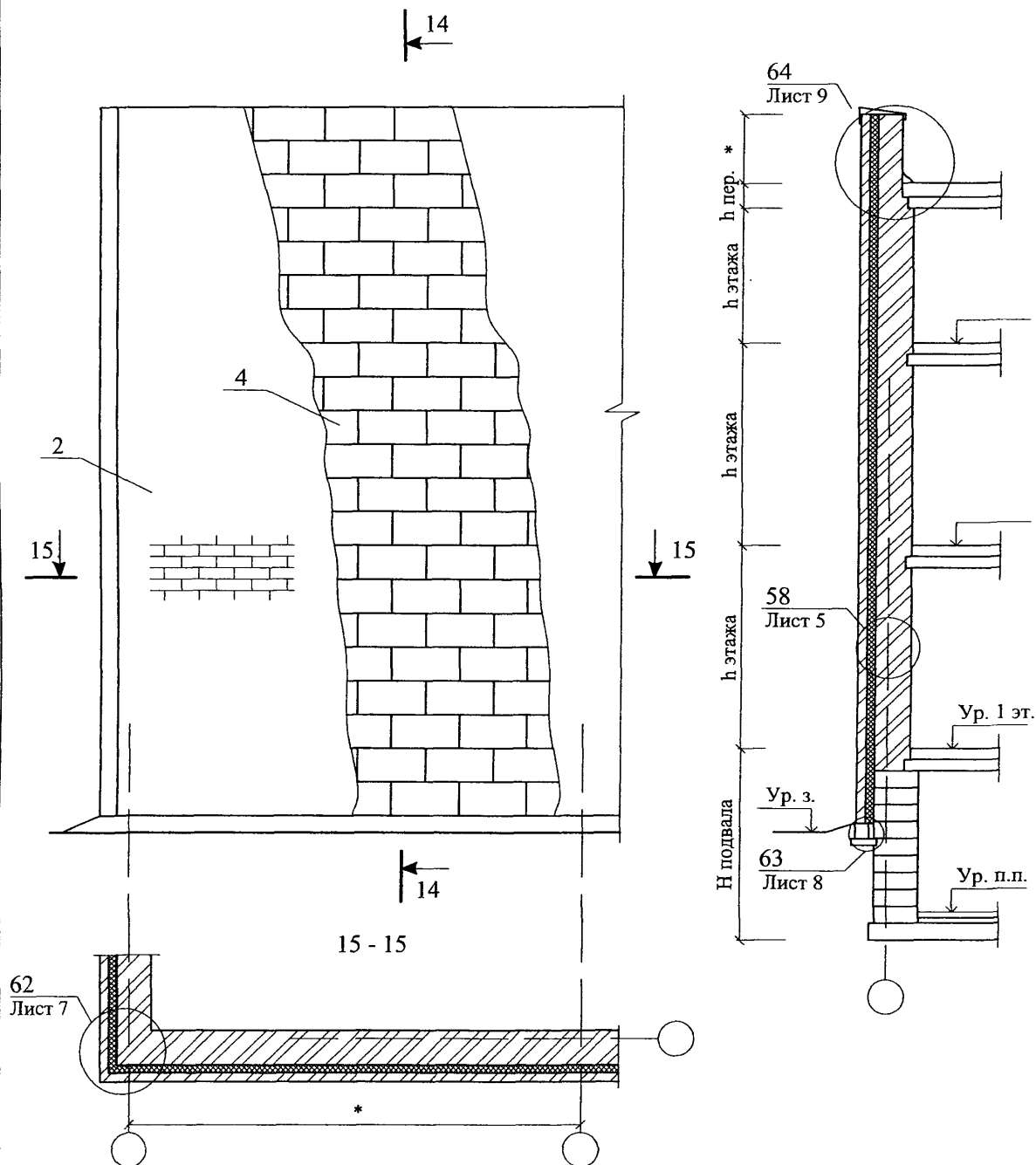
СХЕМА № 11. Расположение плит утеплителя, рассечек
