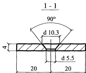
КОСТЫЛЬ К3
